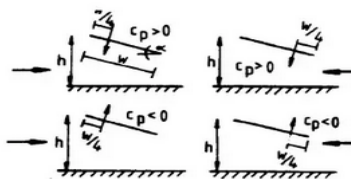
Fig. 10.3.2 – Hipòtesis de carga en marquesinas a un agua
