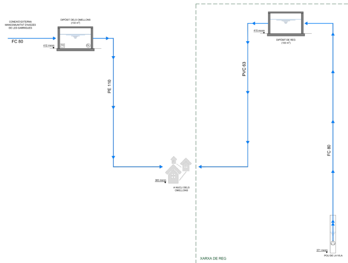
Figura 1: Esquema de la xarxa d'abastament d'aigua potable del municipi dels Omellons
