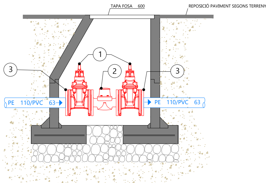
ALÇAT DETALL ARQUETA TIPUS POU
