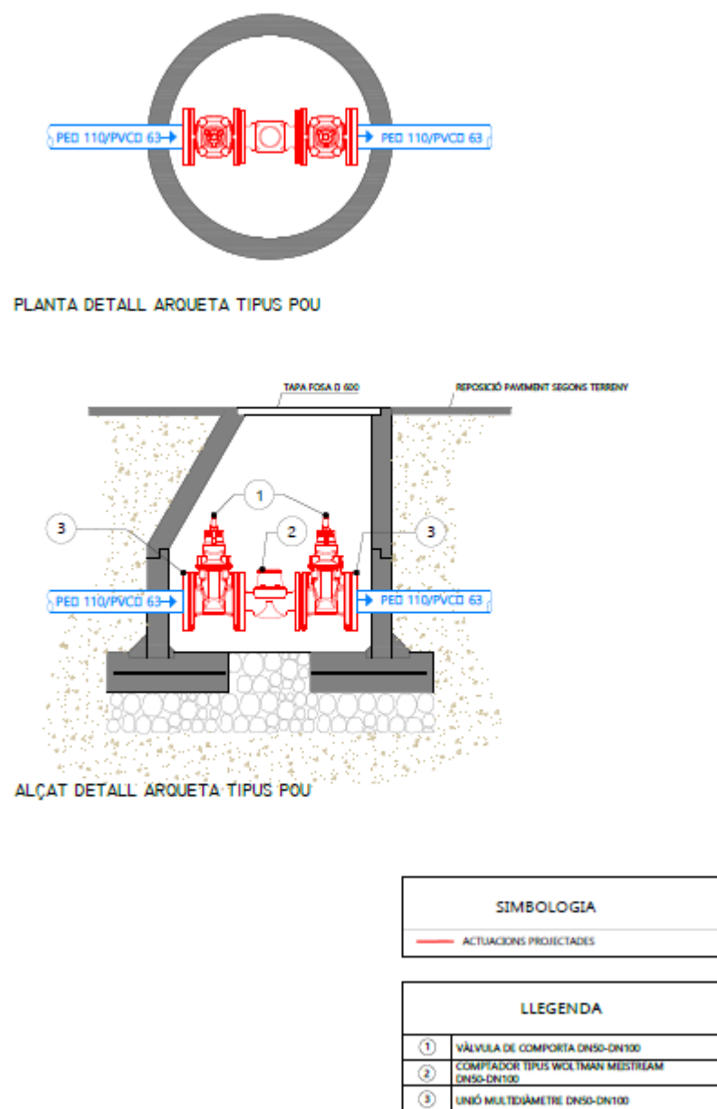
Figura 7: Exemple de disposició dels elements de l'actuació 1: sectorització
