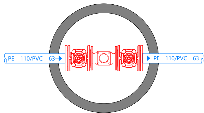
PLANTA DETALL ARQUETA TIPUS POU
