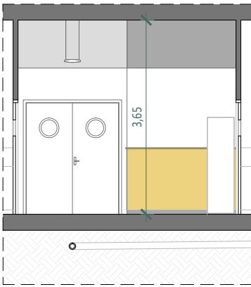
S1 | Secció transversal 1 | e: 1/100
