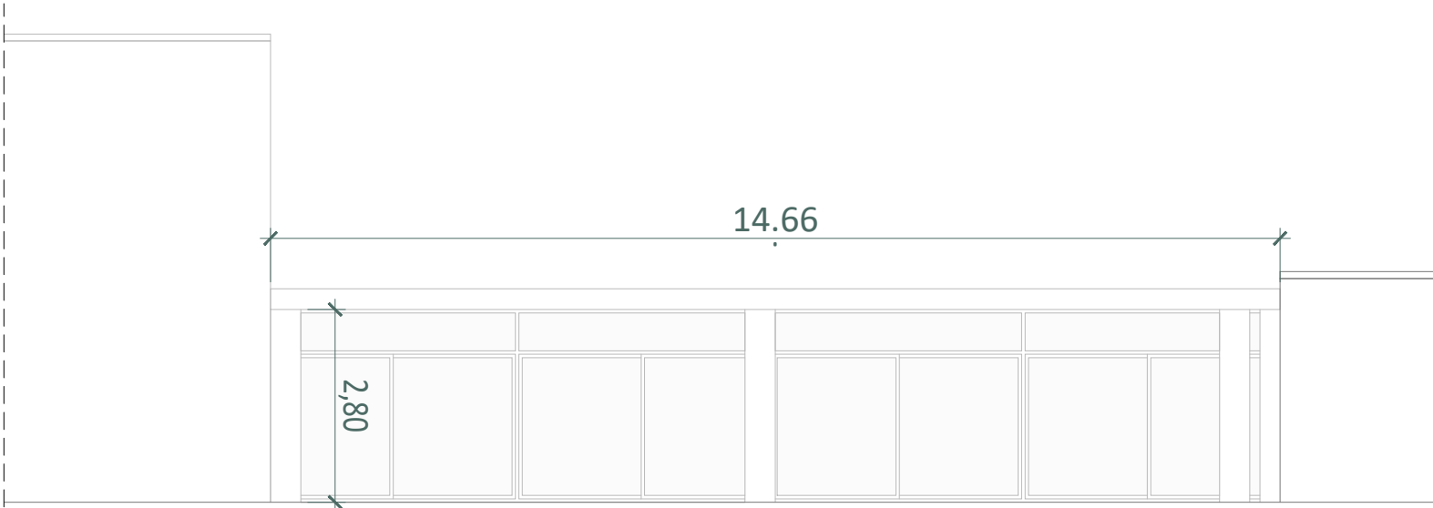
FN.1 | Façana Nord | e: 1/100
