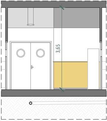
S1 | Secció transversal 1 | e: 1/100
