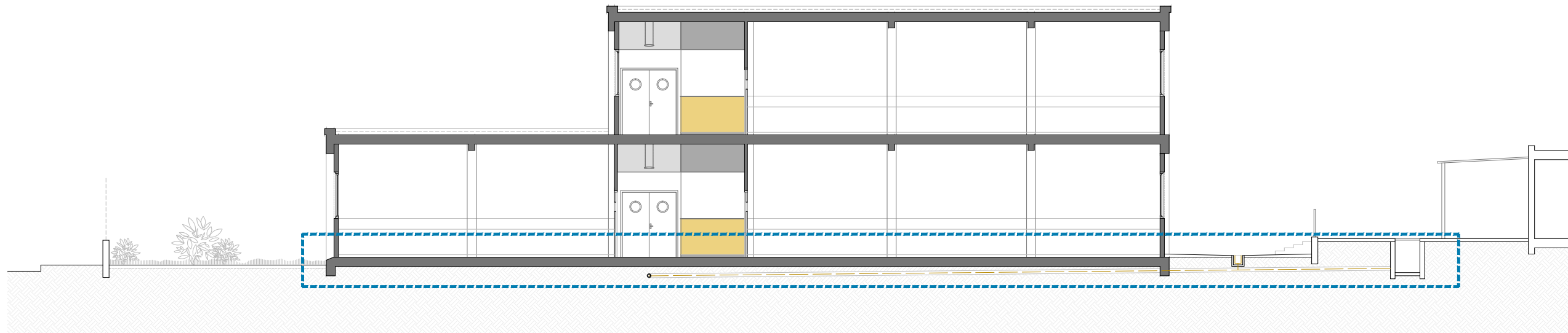
S1 | Secció transversal | e: 1/150
