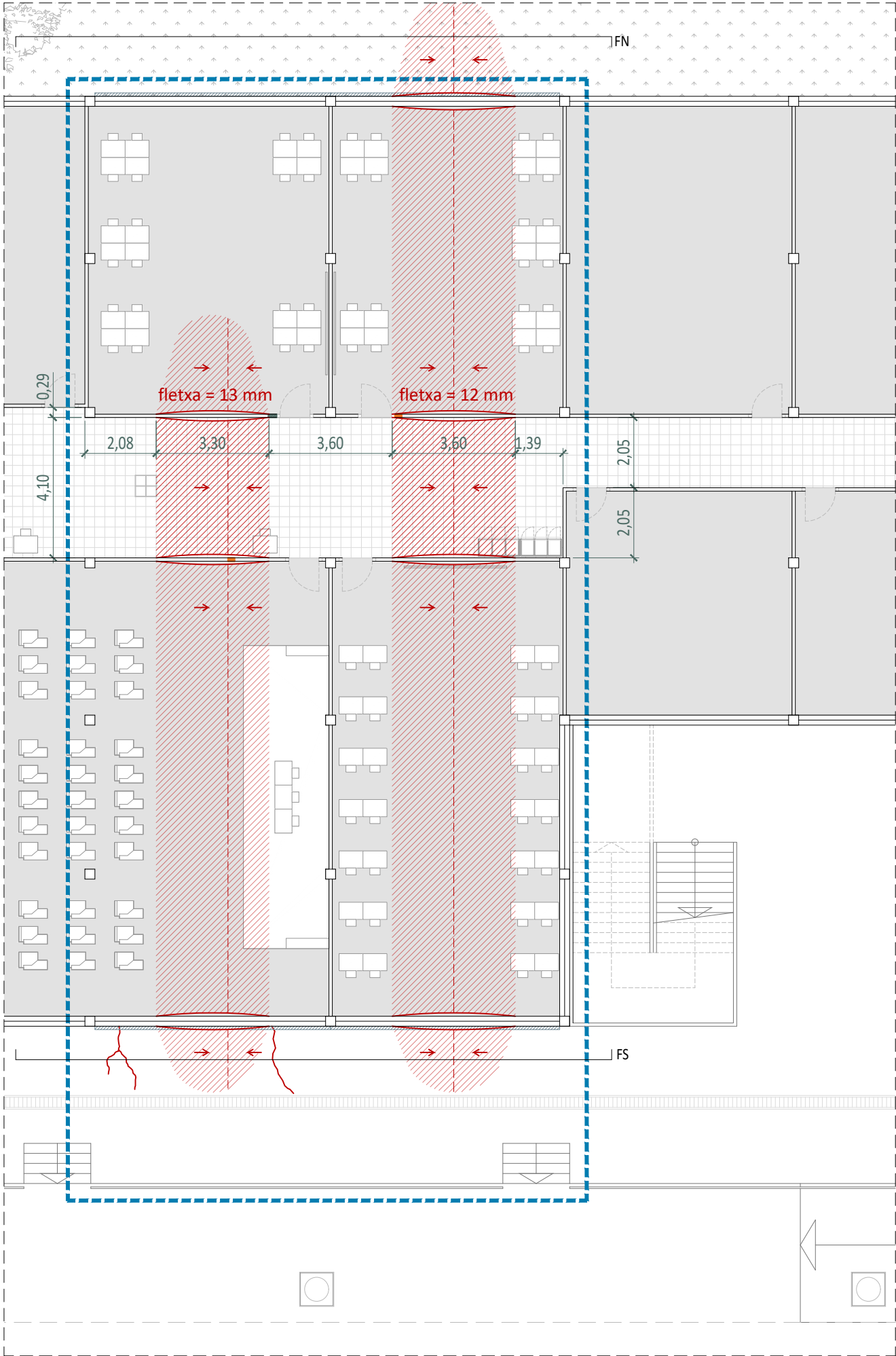
PB | Planta baixa | e: 1/150
