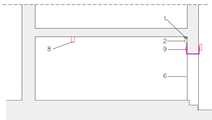
Secció transversal porxo tipus – canalització vista*
