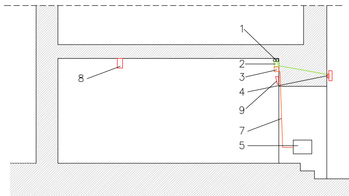
Secció transversal porxo tipus – regata*
