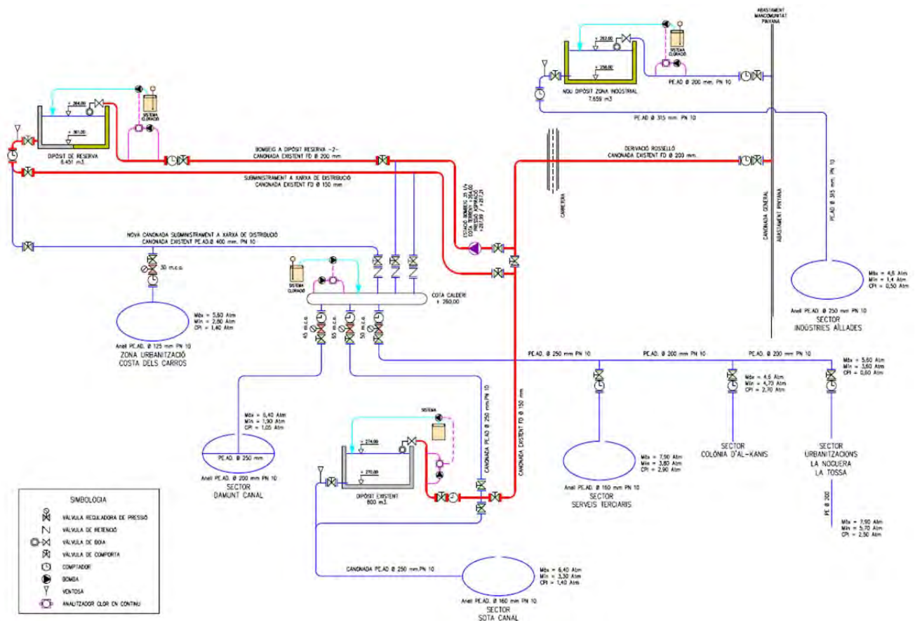
Esquema general d'abastament d'aigua potable. Font: Pla Director d'Abastament d'Aigua de Rosselló
