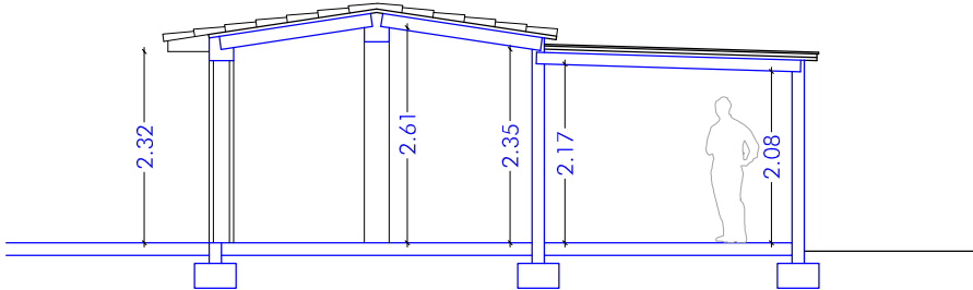
SECCIÓ A
