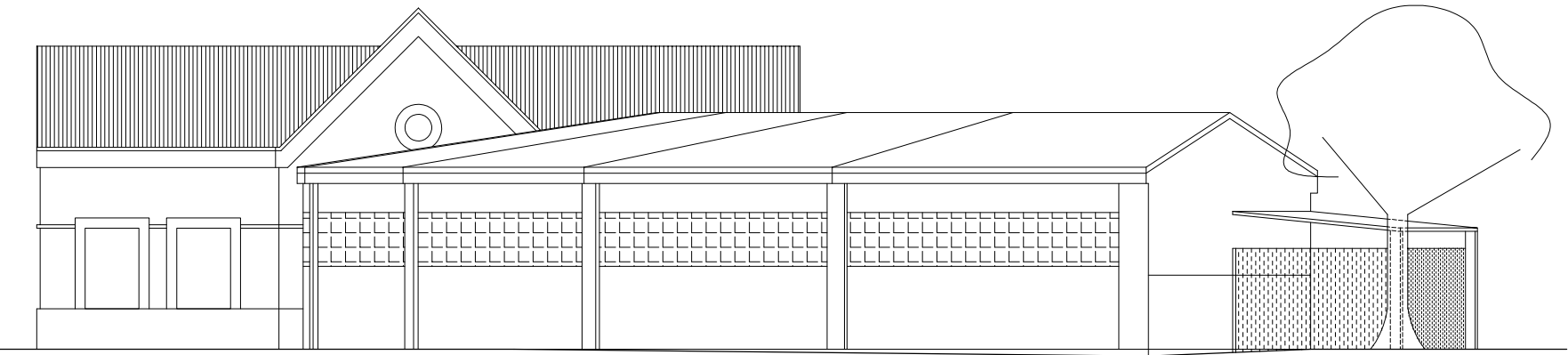
ALÇAT 1
