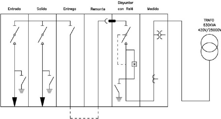
Esquema cel·les actuals
