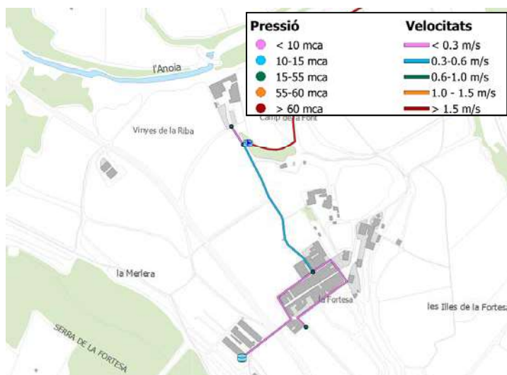
Figura 44. Model de consum de la xarxa actual amb consums punta actuals
