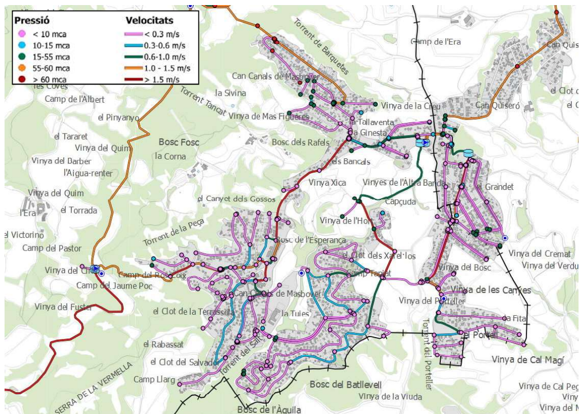
Figura 43. Model de consum de la xarxa actual amb consums punta actuals
