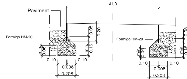
Secció A-A'
