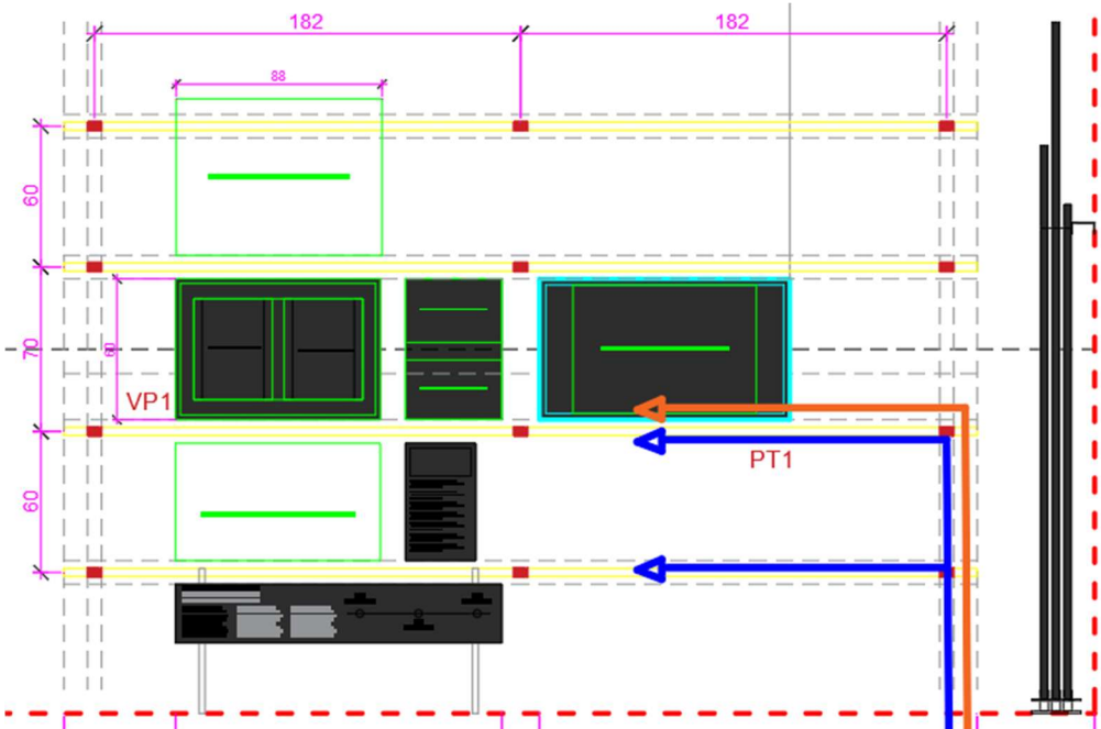
Esquema de cablejat dels monitors de paret
