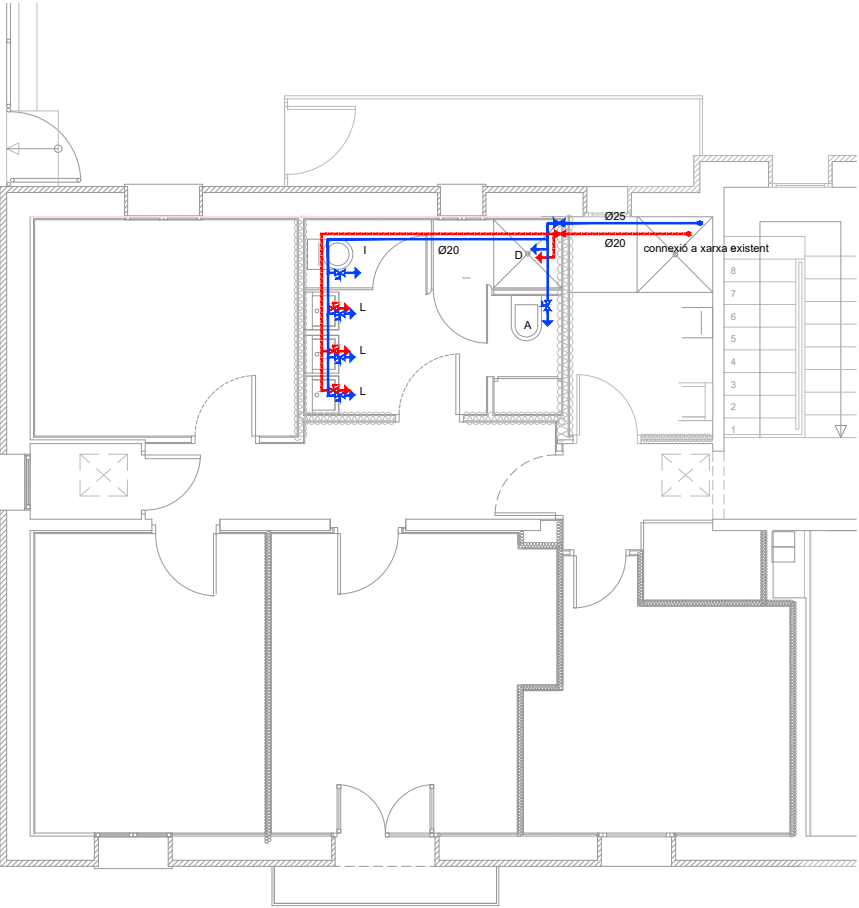
PLANTA BAIXA AIGUA
