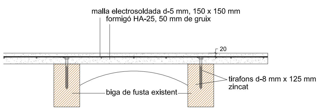
SECCIÓ TRANSVERSAL
