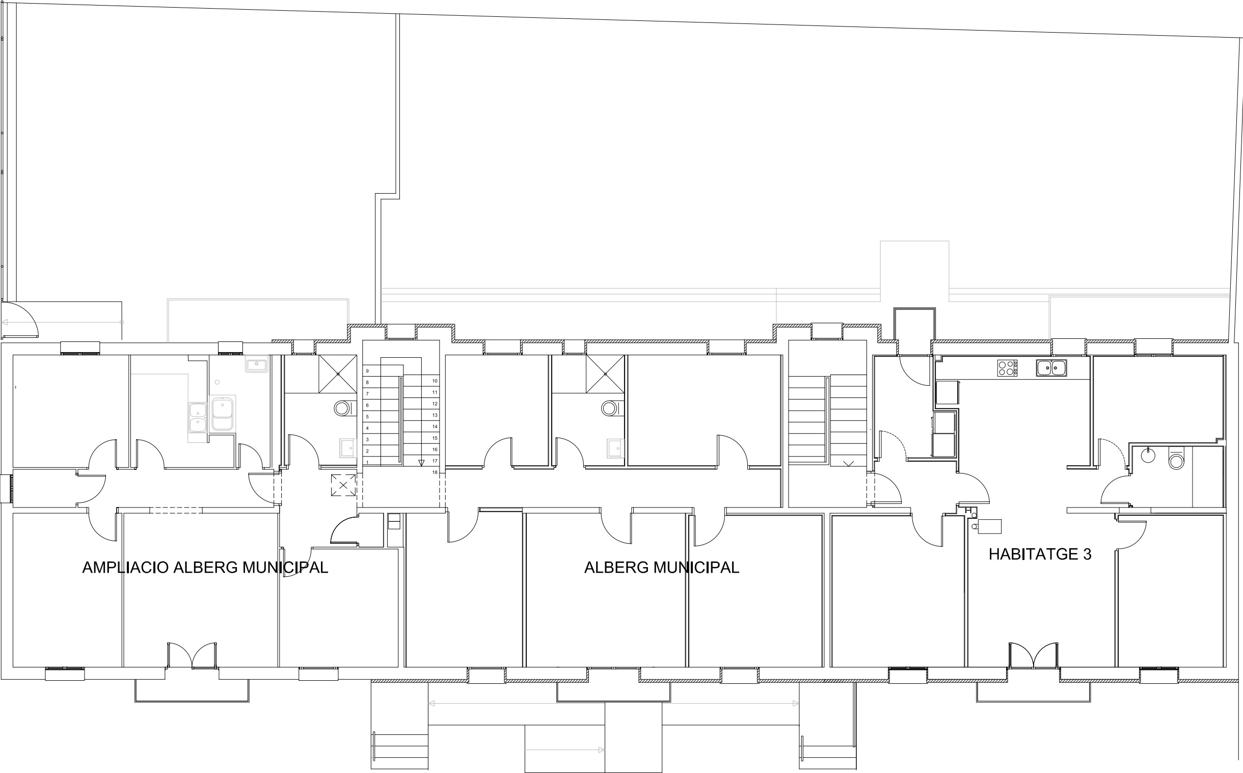
PLANTA PIS HABITATGE 3
