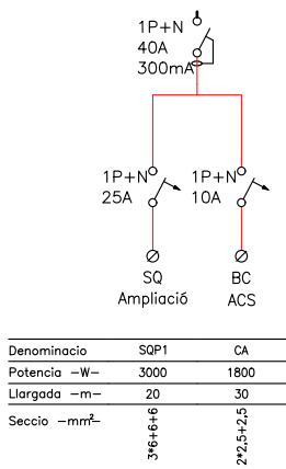
AMPLIACIÓ EN QUADRE GENERAL
