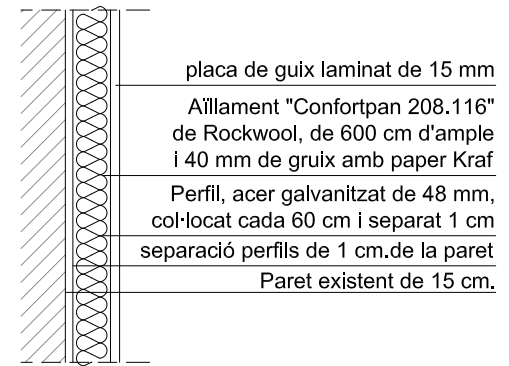
DETALL T-01 E: 1/10
