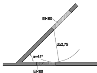
Figura 1.2. Fachadas a 45°
