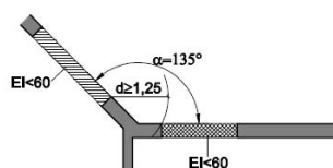
Figura 1.5. Fachadas a 135°
