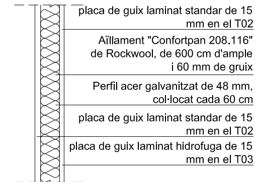
DETALL T-02 i T-03 E: 1/10
