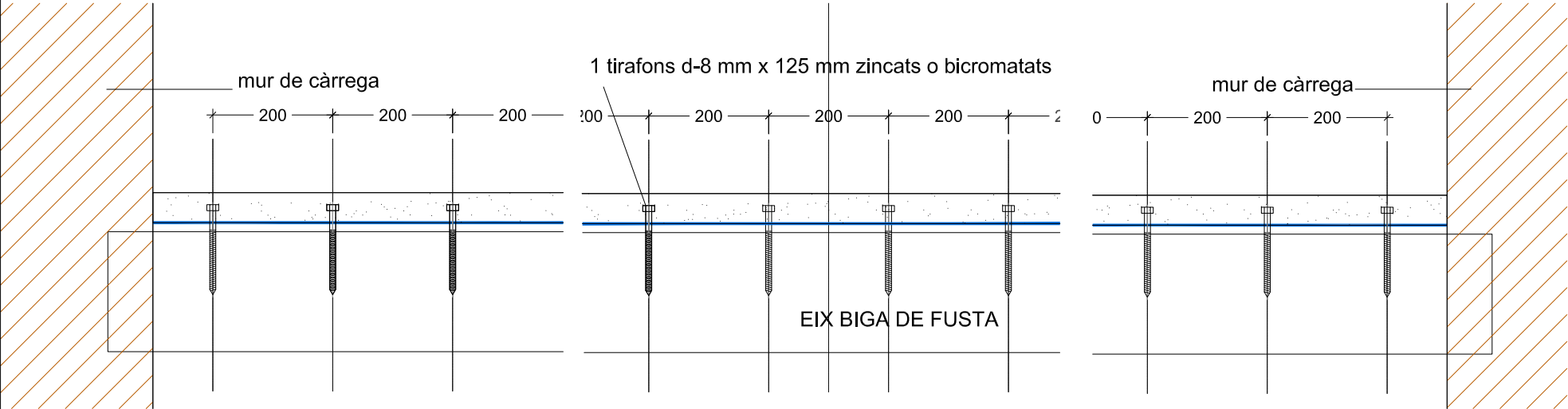
SECCIÓ LONGITUDINAL AMB DISTRIBUCIÓ DELS TIRAFONS CONECTORS
