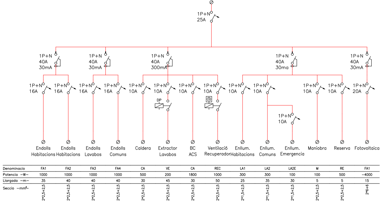
SQ-AMPLIACIÓ
