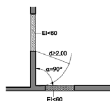
Figura 1.4. Fachadas a 90°
