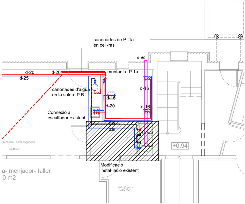
PLANTA BAIXA AIGUA
