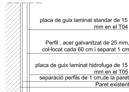
DETALL T-04 i T-05 E: 1/10
