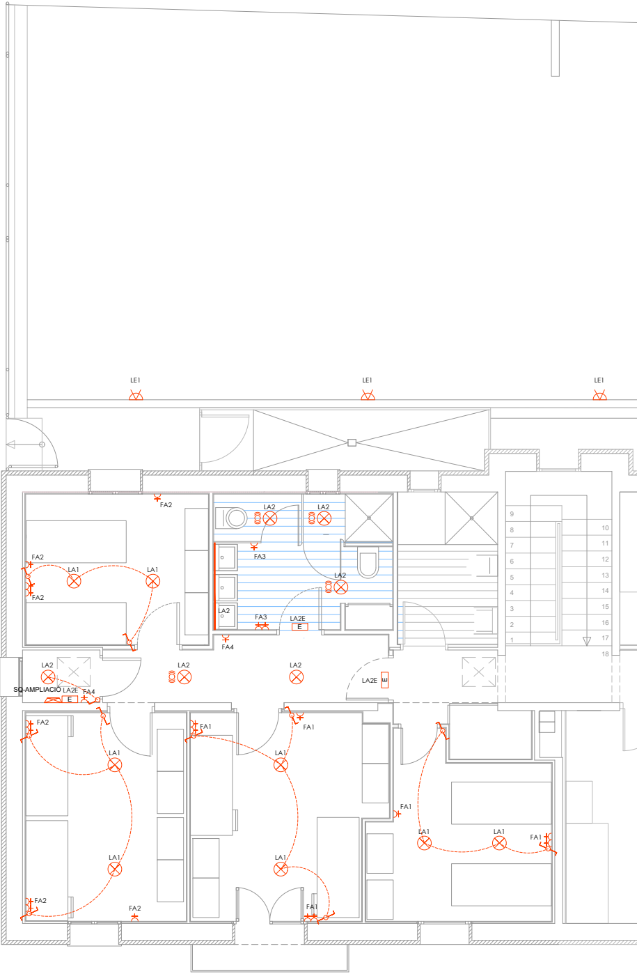
PLANTA PRIMERA ELECTRICITAT
