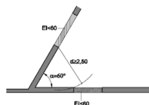
Figura 1.3. Fachadas a 60°
