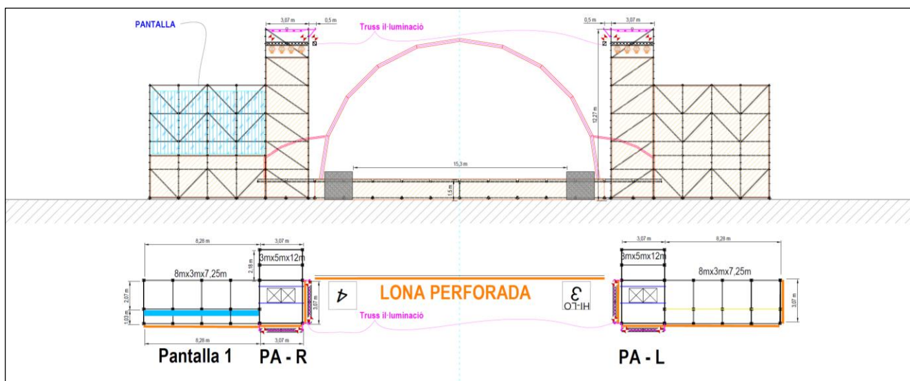
Vista frontal i planta torres de PA
