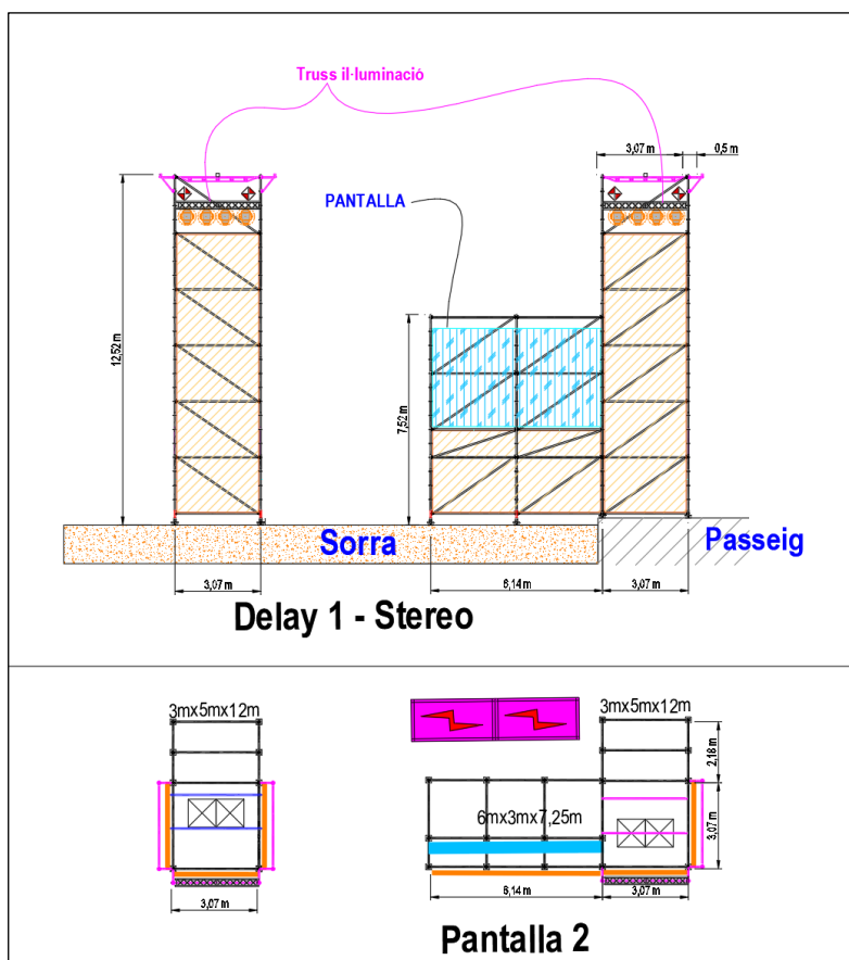
Vista frontal i planta Delay 1
