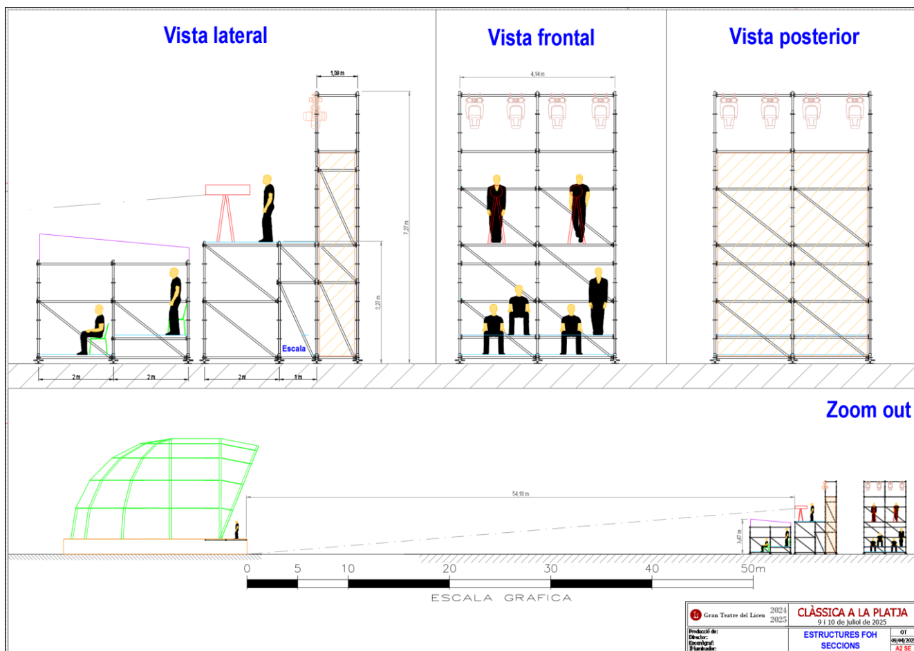
Plànol i secció Control i FOH
