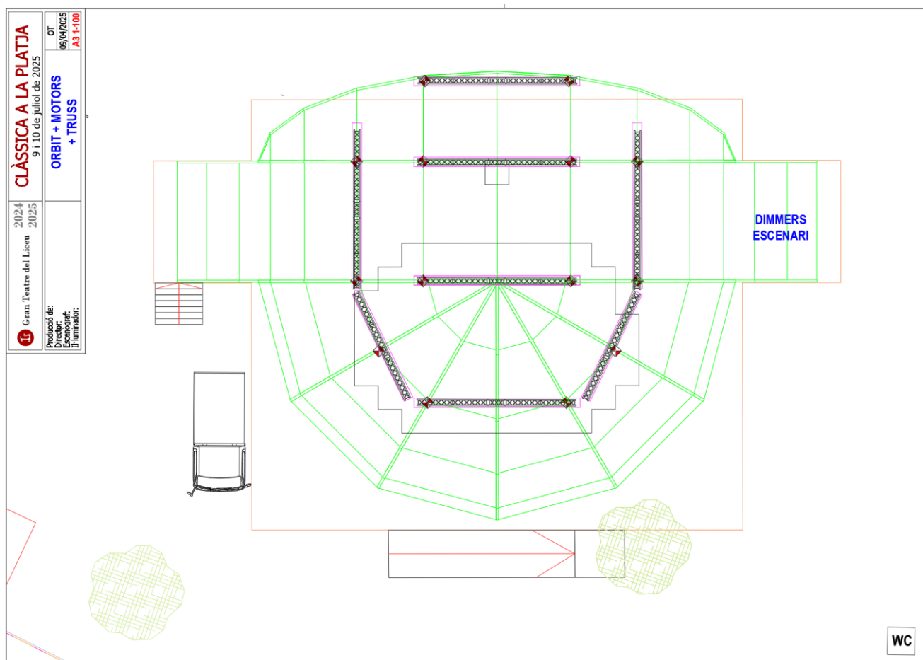
Plànol preliminar de l'escenari, motors i truss.
