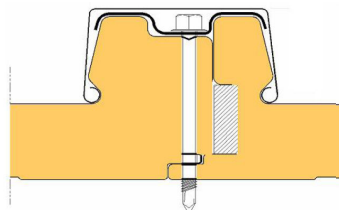
Sección Machihembrado (fija. oculta)
