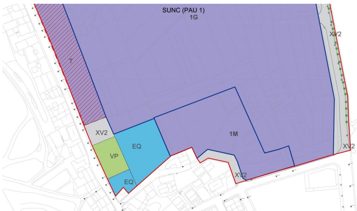
Fragment del plànol d'ordenació O.4. de la MP del POUM (any 2023).
