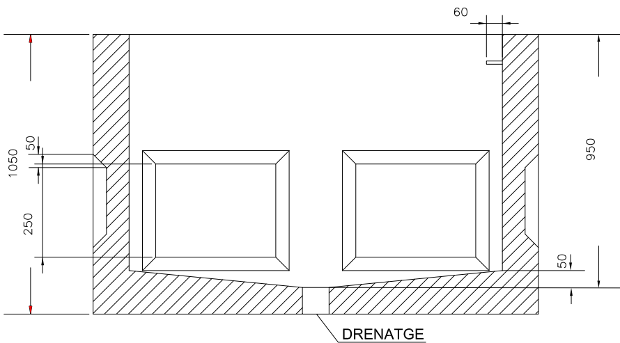
SECCIÓ C-D
