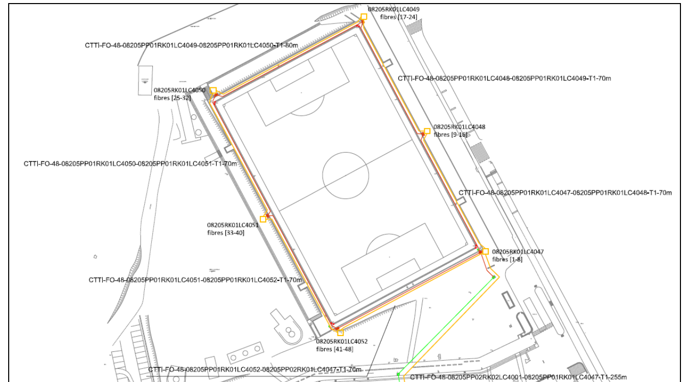
Plànol d'estesa del cable de 48FO i assignació de fibres per nova canalització al voltant del camp de futbol passant pels 6 armaris d'exterior a instal·lar (Capítol 2.5 Plànols de Detall d'estesa de fibra òptica)
