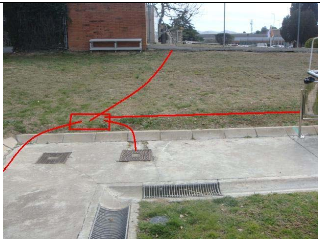
Ubicació del 1er armari 08205RK01LC4047 amb la canalització que arriba des del pericó 08205PE0985, la connexió a l'arqueta elèctrica i les canalització amb micro-rasa que surten cap als armaris segon i sisè
