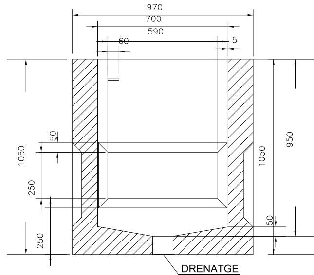
SECCIÓ E-F
