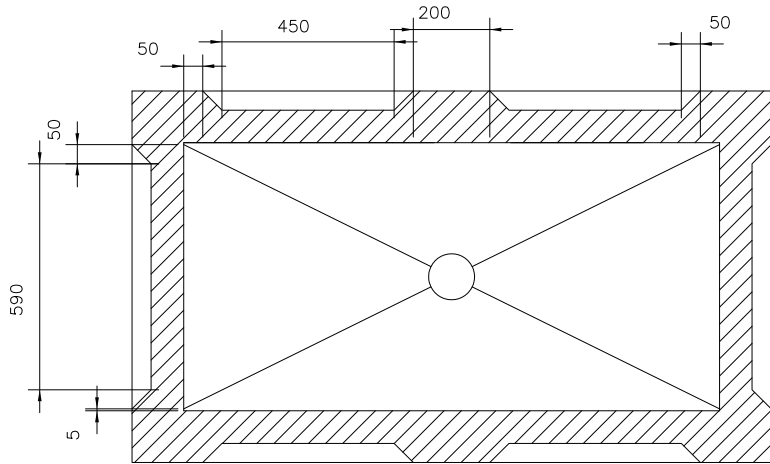
SECCIÓ A-B
