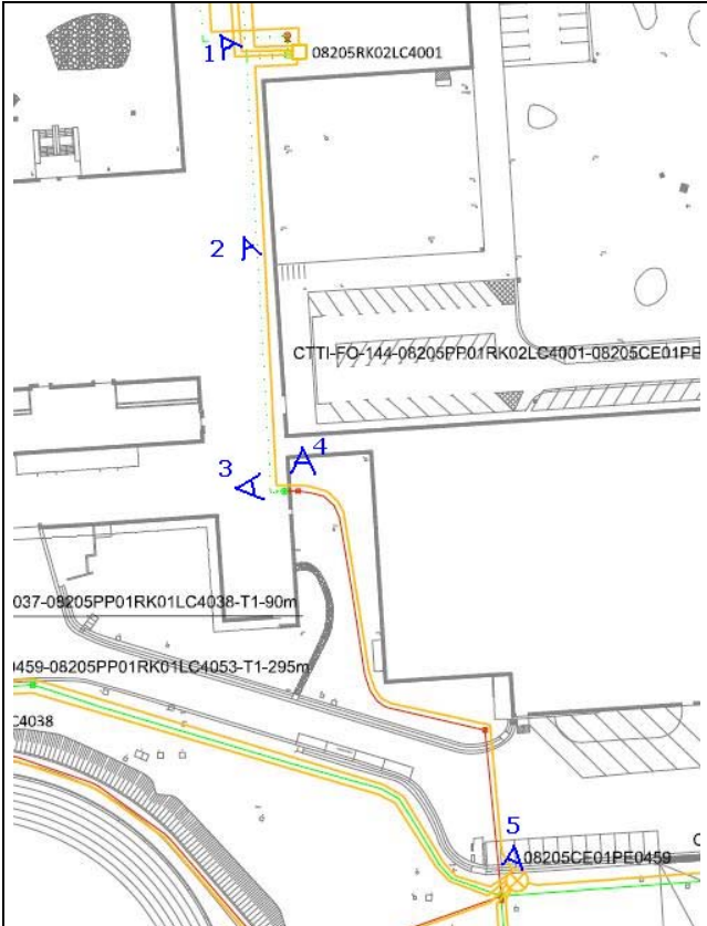
Plànol del traçat del cable de 144 FO des del NCC fins al pericó 08205PE0459 (Capítol 2.5 Plànols de Detall d'estesa de fibra òptica)
