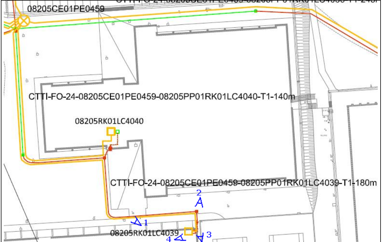
Plànol d'estesa del cable de 24 FO des de la caixa d'empalme 08205CE01PE0459 fins al rack del mòdul d'atletisme 08205RK01LC4039 (Capítol 2.5 Plànols de Detall d'estesa de fibra òptica)
