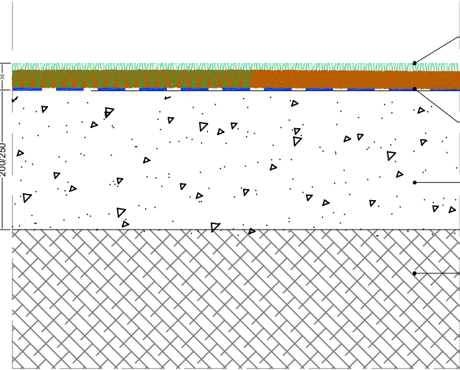
SECCIÓ-DETALL CONJUNT BASE-GESPA ARTIFICIAL
