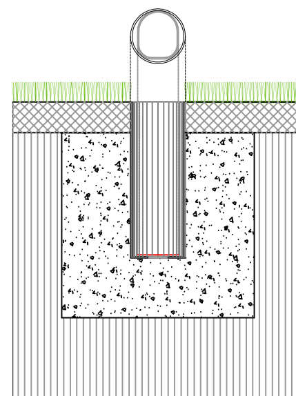
DETALL BEINES DE TUB D'ACER GALVANITZAT
