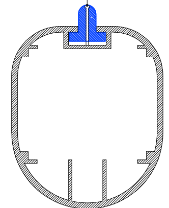
DETALL PERFIL D'ALUMINI DE POSTES I TRAVESSER
