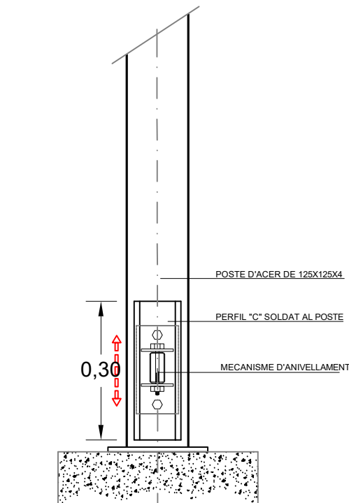
DETALL DEL MECANISME D'ANIVELLAMENT DEL BRAÇ TELESCÒPIC GIRATORI
