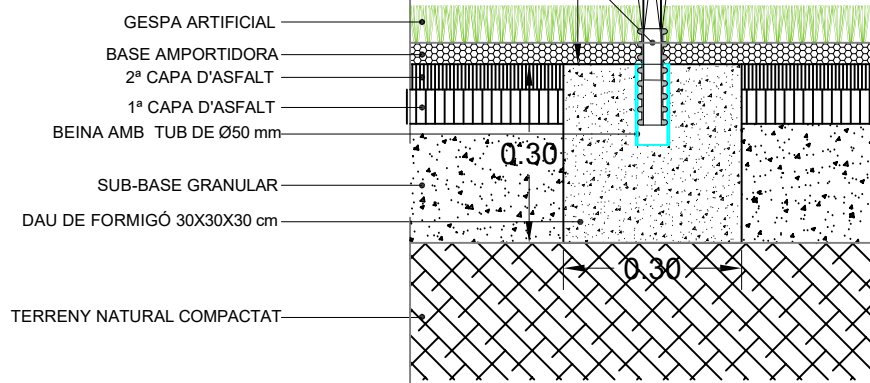
DETALL DE L'ANCORATGE DELS BANDERINES
