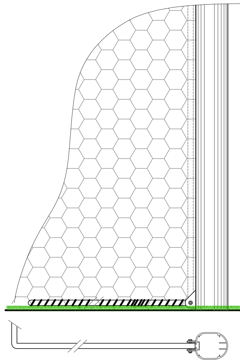
DETALL DE LA FIXACIÓ DE LA BARRA D'ANCORATGE INFERIOR DE LES XARXES AMB ELS POSTES DE LA PORTERÍA
