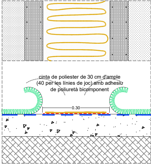
DETALL DE L'ENCOLAT DE LES JUNTES I LÍNIES DE JOC
