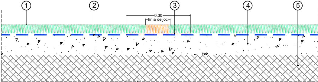
SECCIÓ-DETALL INSERCIÓ LÍNIES DE JOC (8 cms d'ample per futbol sala)
