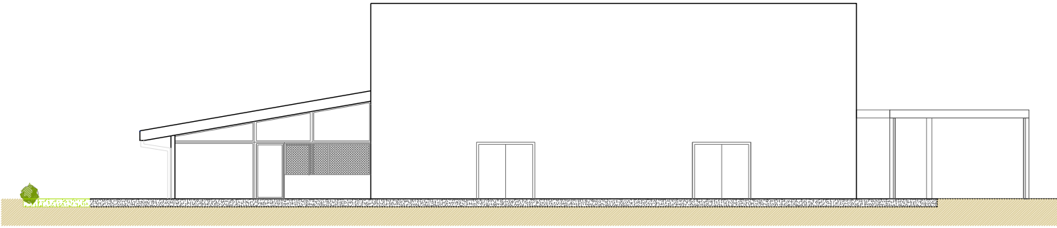
A2. Alçat Nord
