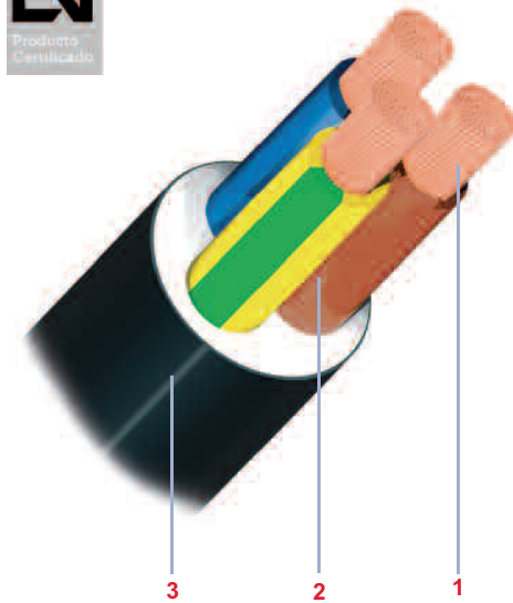
Simulación Cable RV-K 0.6/1 kV 3G10 mm²
