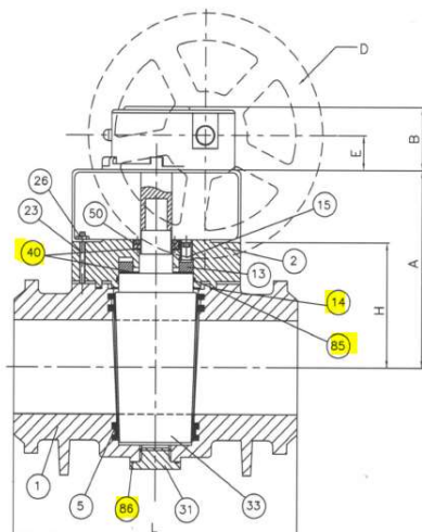
Vàlvula mascle MTS flushing DN80
