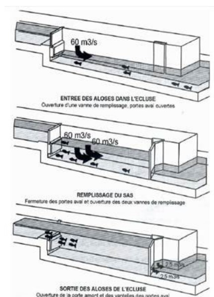
Figura 1. Visió esquemàtica de les fases de funcionament de les resclosos per a navegació adaptades a les necessitats de migració de la saboga (Alosa fallax) al tram inferior del riu Roine (França). Font: Association Migrateurs du Rhône-Méditerranée (2007), a partir de Bechu et al. (1995).
