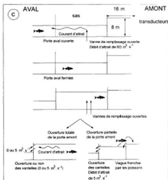
Figura 2. Esquema del funcionament de la resclosa per a navegació adaptada a les necessitats de migració de la saboga (Alosa fallax) a Beucauire-Vallagrègues, al tram inferior del riu Roine (França). Font: Guillard & Colon (1998).
