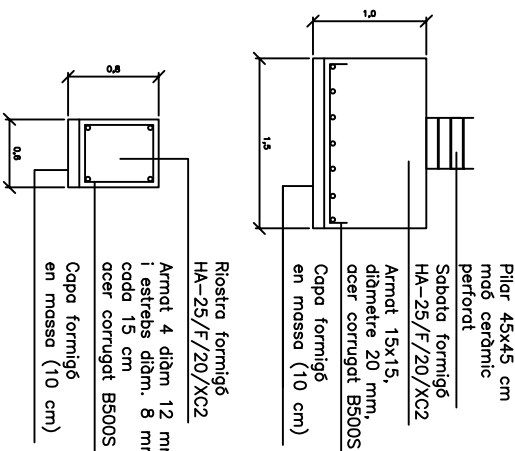
DEALLS FONAMENTACIÓ
