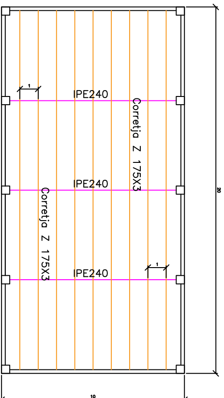
PLANTA ESTRUCTURA
