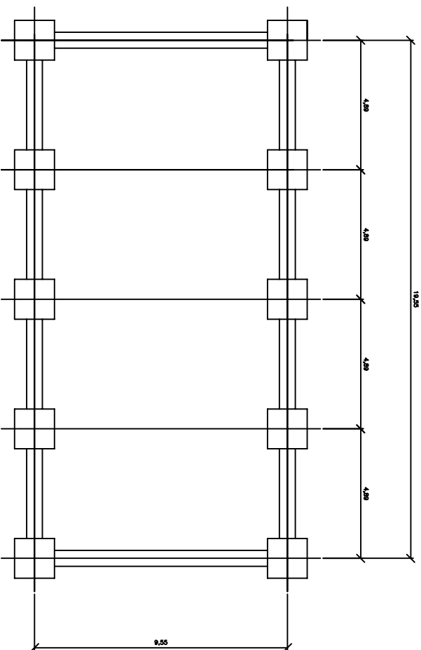
PLANTA FONAMENTACIÓ
