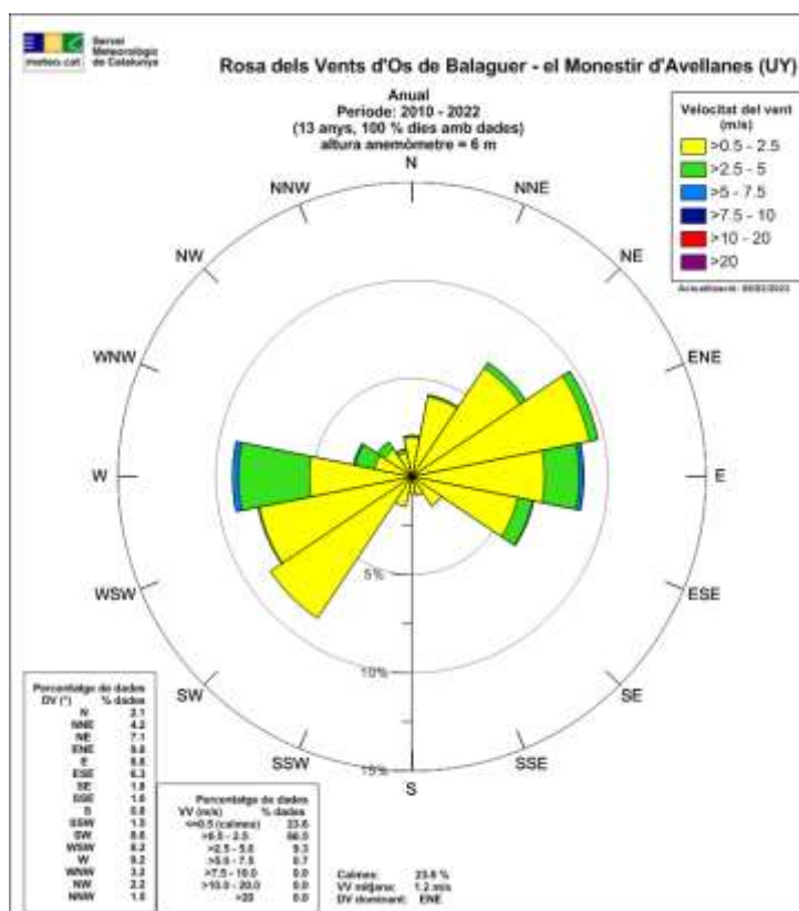
Figura 5. Rosa dels vents a Os de Balaguer – Monestir de les Avellanès. Font: Servei Meteorològic de Catalunya .
