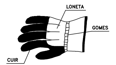
GUANTS DE PROTECCIÓ CONTRA RISCOS MECÀNICS
