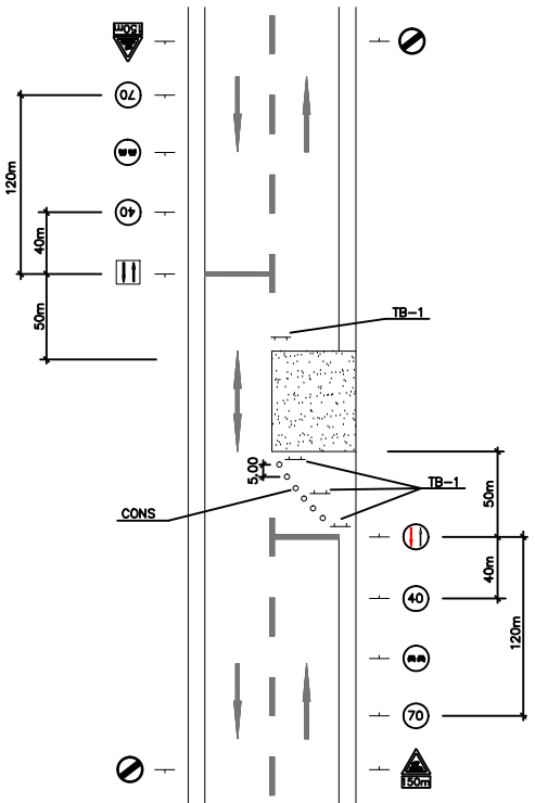
OBRES QUE OCUPEN UNA VIA COMPLETA.
