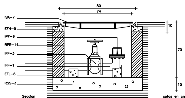
Seccion
