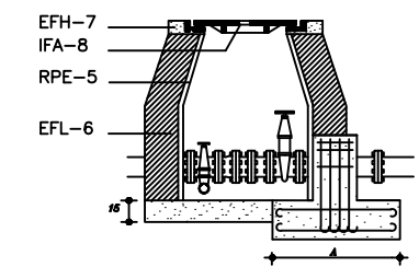
Seccion
