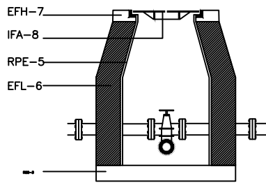
Seccion
