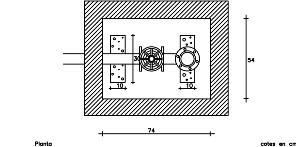
Planta
