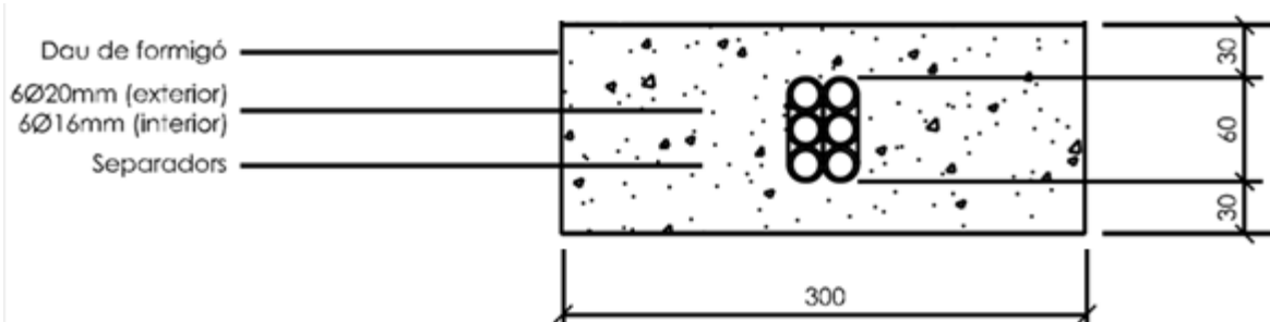
Detall de canalització amb 2 tritubs sota nova cuneta
