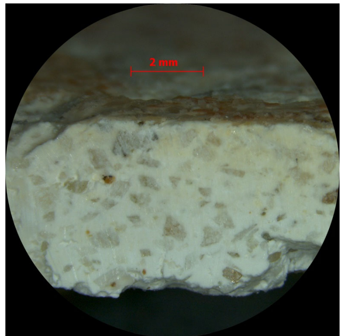
Micrografia de l'arrambador marbrejat original del vestíbul: Estuc de calç acabat acolorit amb els tons G/H/I.
