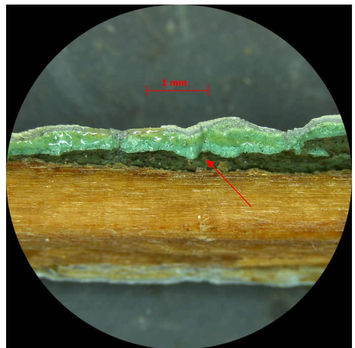
Estratigrafia de les finestres del pati a 16X: En contacte amb la fusta es detecta l'acabat més antic corresponent amb el Color E.
