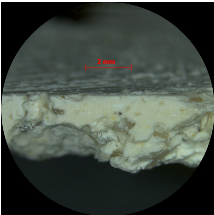
Micrografia del parament original del vestíbul: Estuc tradicional de calç acabat lliscat i del Color E, amb repintat antic.
