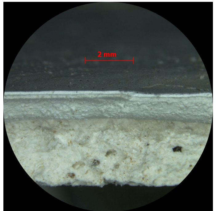
Micrografia de l'arrambador de l'escala en el 1er tram: comparat amb la micrografia anterior s'observa un morter de guix repintat corresponent a una reparació moderna.
