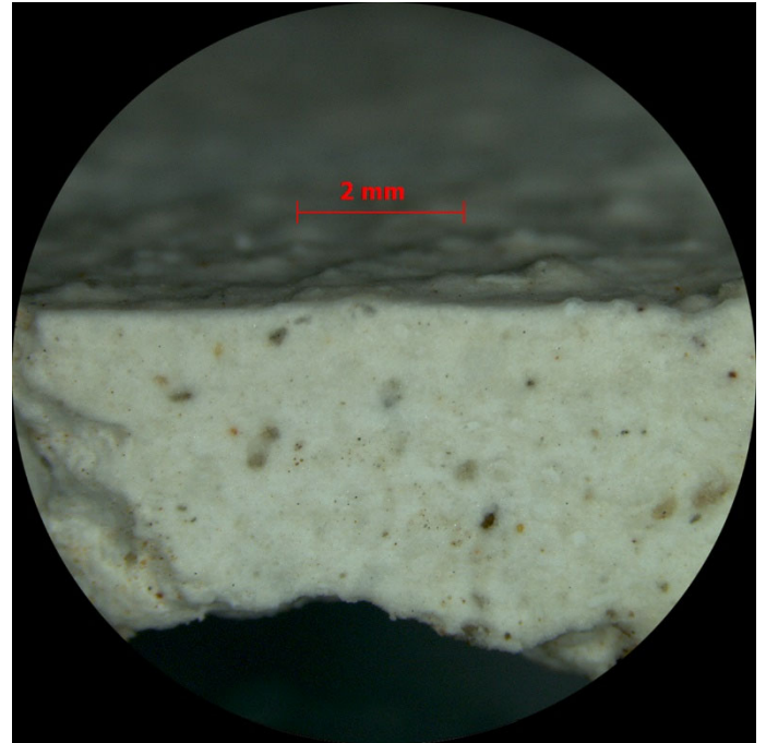
Micrografia del parament del 1er tram d'escala: en la comparativa amb la micrografia anterior es pot apreciar que es tracta d'un enguixat repintat fruit d'una intervenció de substitució moderna.
