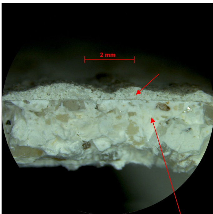
Micrografia del parament del pati interior: Estuc de calç lliscat del Color D, actualment repintat amb pintura texturada blanca tipus "gotelé".
