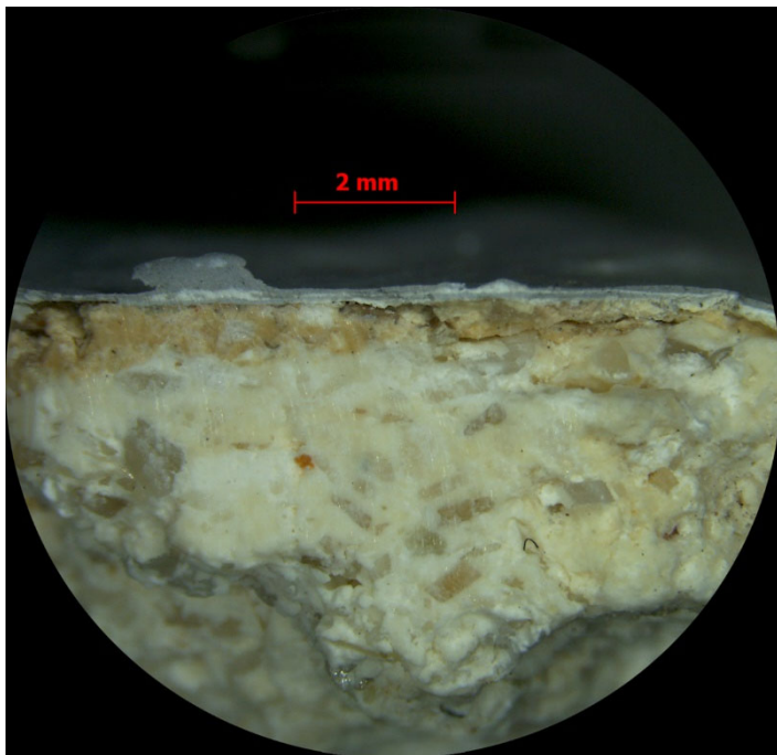
Micrografia de l'arrambador original de l'escala: estuc de calç pigmentat i acabat del Color G com a fons del marbrejat, sobre el qual es detecten repintats filmògens com l'esmalt gris actual.
