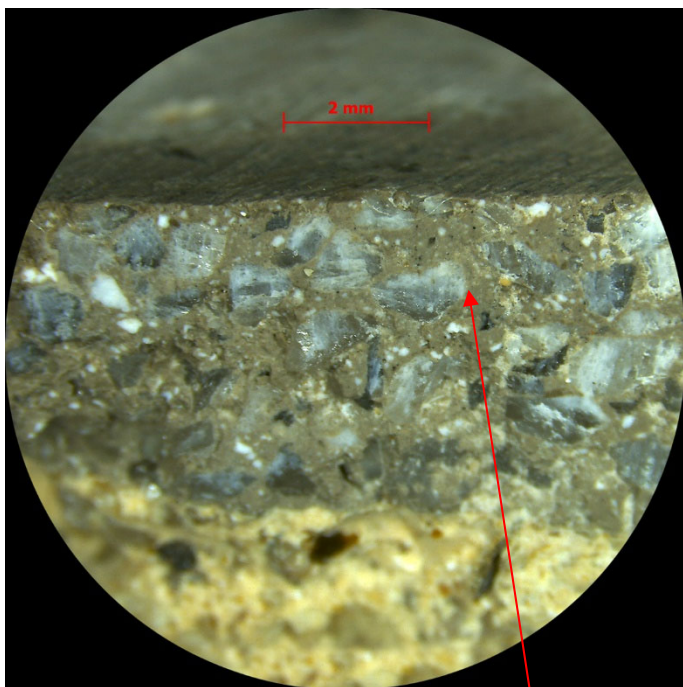
Micrografia del parament de façana: Estuc de calç pigmentat en massa que en textura desbastada té el Color A mentre que en textura lliscada és del Color B.
