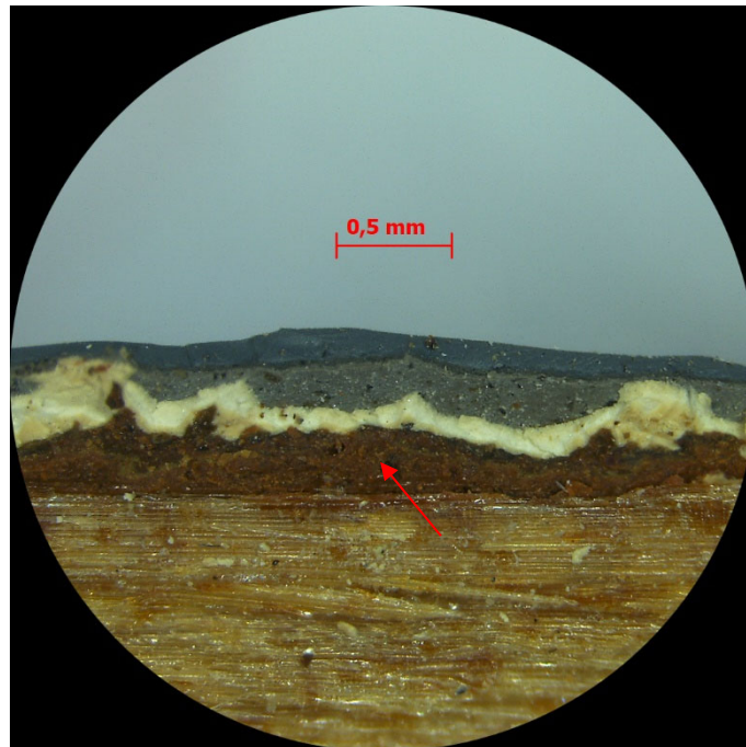
Micrografia de les balconeres de façana a 25X: S'observen tots els estrats dels diferents esmalts, detectant com l'acabat més antic el del Color C.
