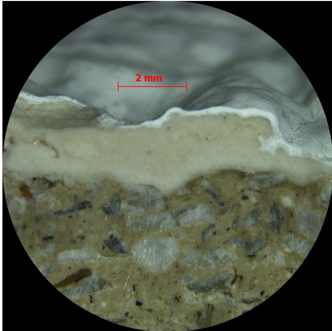
Micrografia del parament original de l'escala: Estuc tradicional de calç pigmentat en massa del Color J, amb el repintat texturat al damunt.
