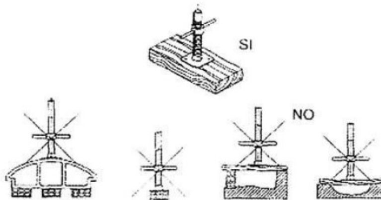
Figura 1. Suport correcte i incorrecte de les bastides
