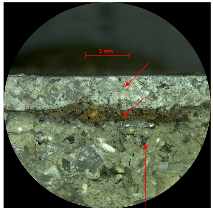
Micrografia del parament de pl. baixa: Comparada amb la mostra anterior, és el mateix estuc que al damunt presenta una reparació de morter sobre brutícia.
