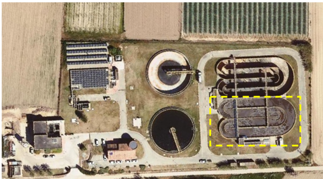
Figura 2. Ubicació de l'aeració de la línia 1 de l'EDAR de Torroella de Montgrí.
