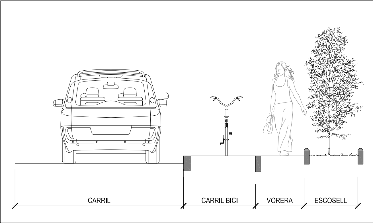
SECCIO TIPUS
