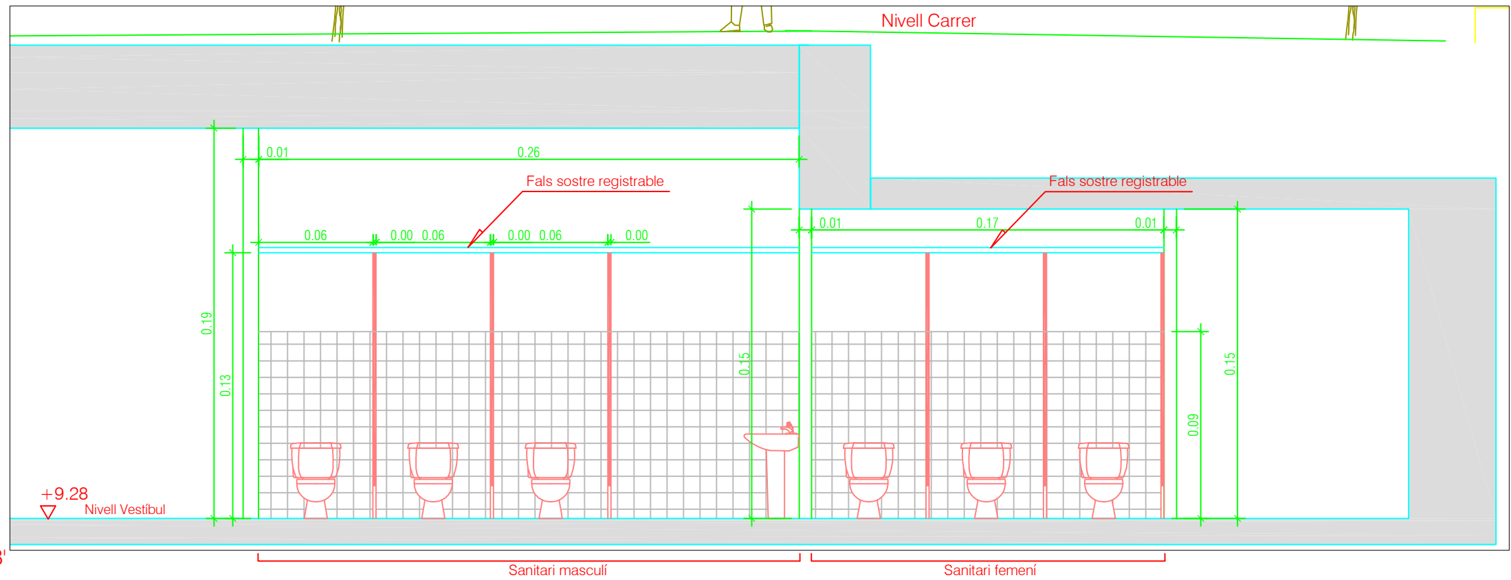
Secció longitudinal B-B' Escala 1:50
