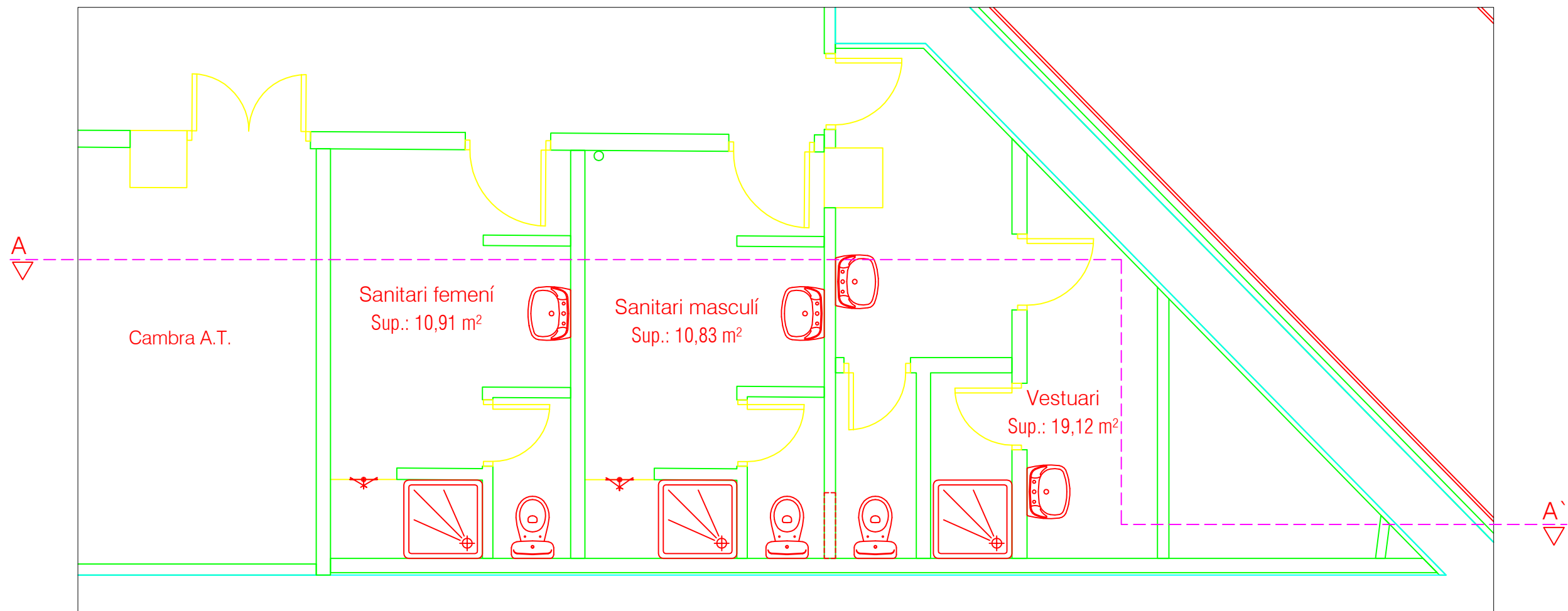
Planta distribució (actual) Escala 1:50
