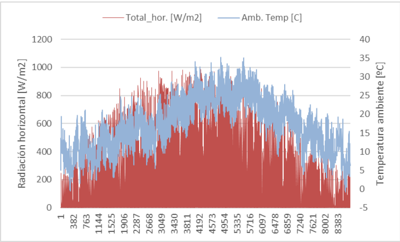
Figura 8. Radiació solar horitzontal i temperatura ambient [METEONORM].
