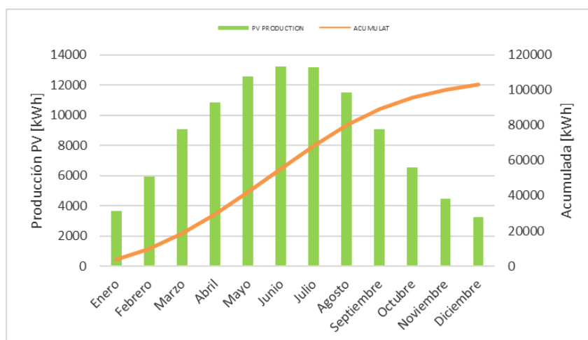
Figura 5. Producció mensual i anual d'electricitat de la instal·lació projectada.
