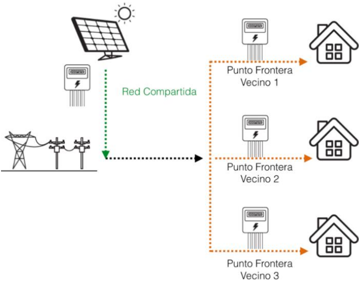
Figura 6. Esquema de funcionament d'una instal·lació fotovoltaica compartida connectada a la xarxa interior amb venda/compensació d'excedents.
