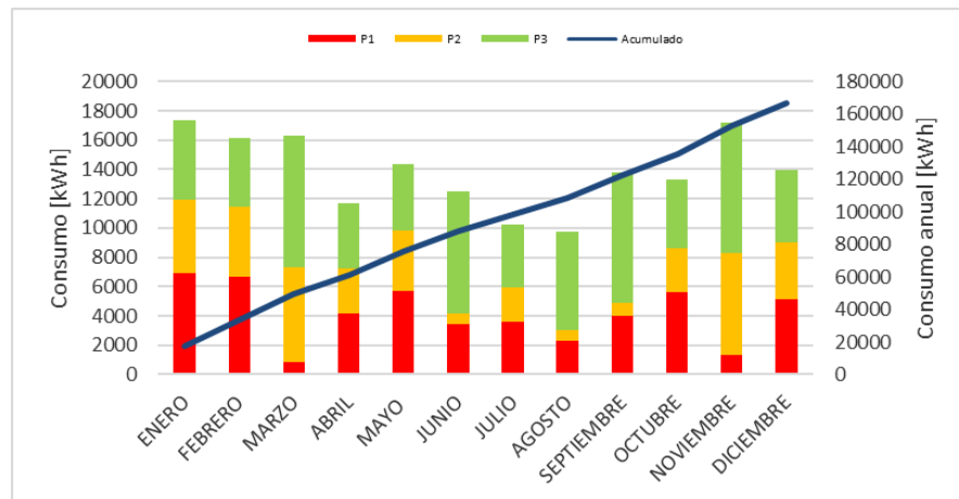
Figura 4. Consum energètic mensual i anual dels consums actuals.
