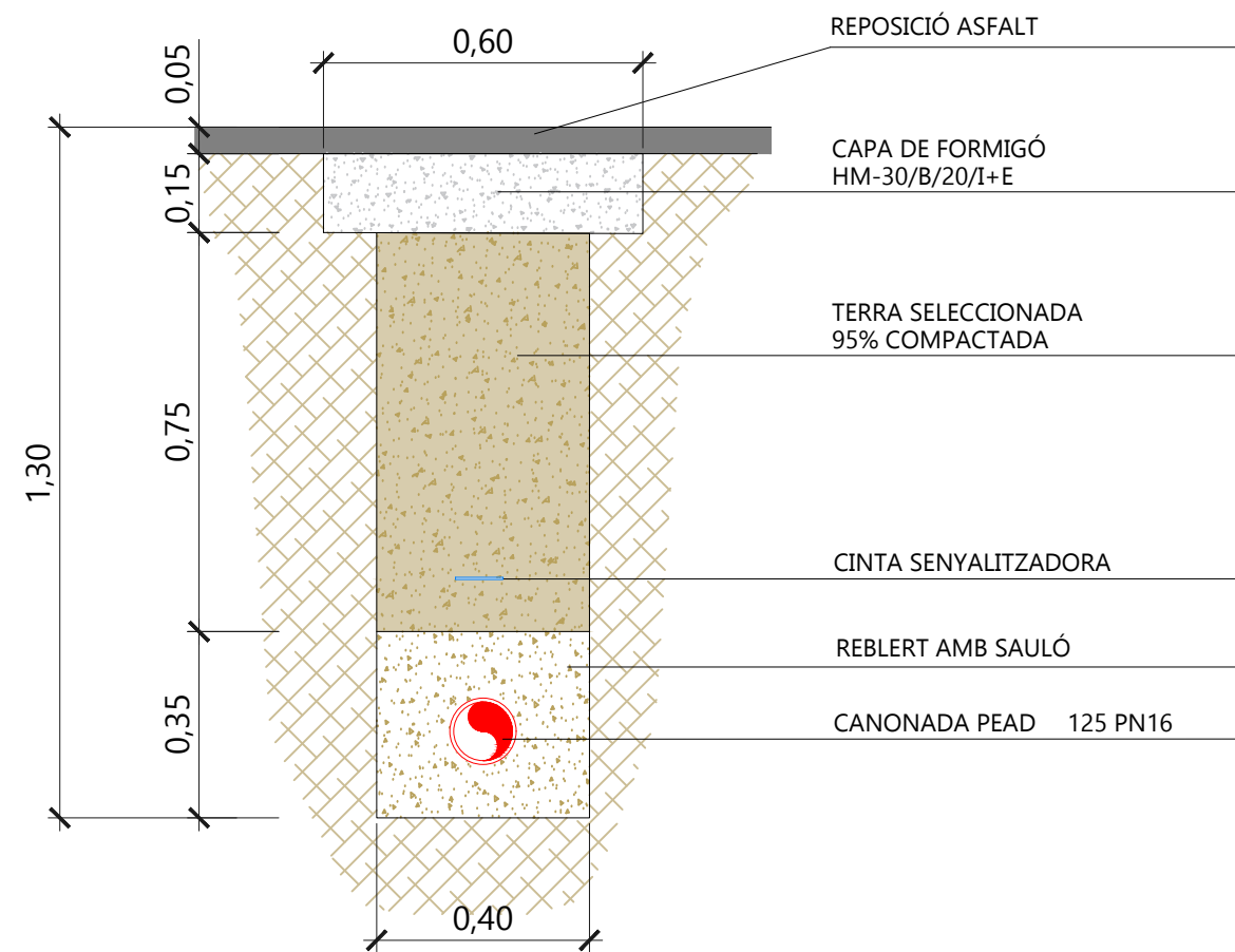
DETALL RASA SECCIÓ PAVIMENT ASFALT ESCALA 1:15
