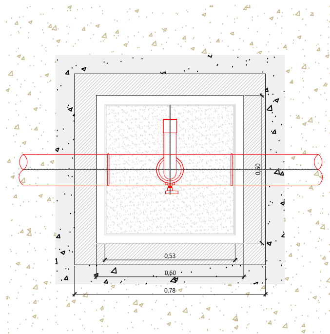
DETALL PLANTA ARQUETA AMB VENTOSA ESCALA 1.15
