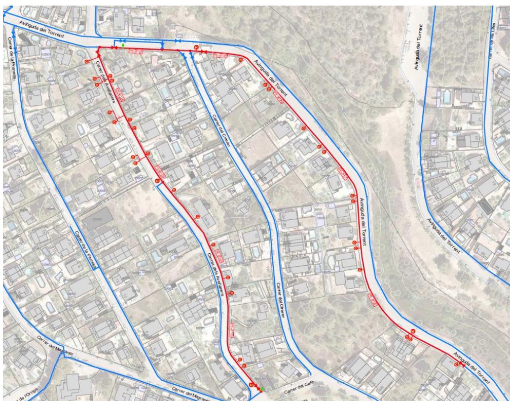
Figura 1. Traçat de canonada projectada
