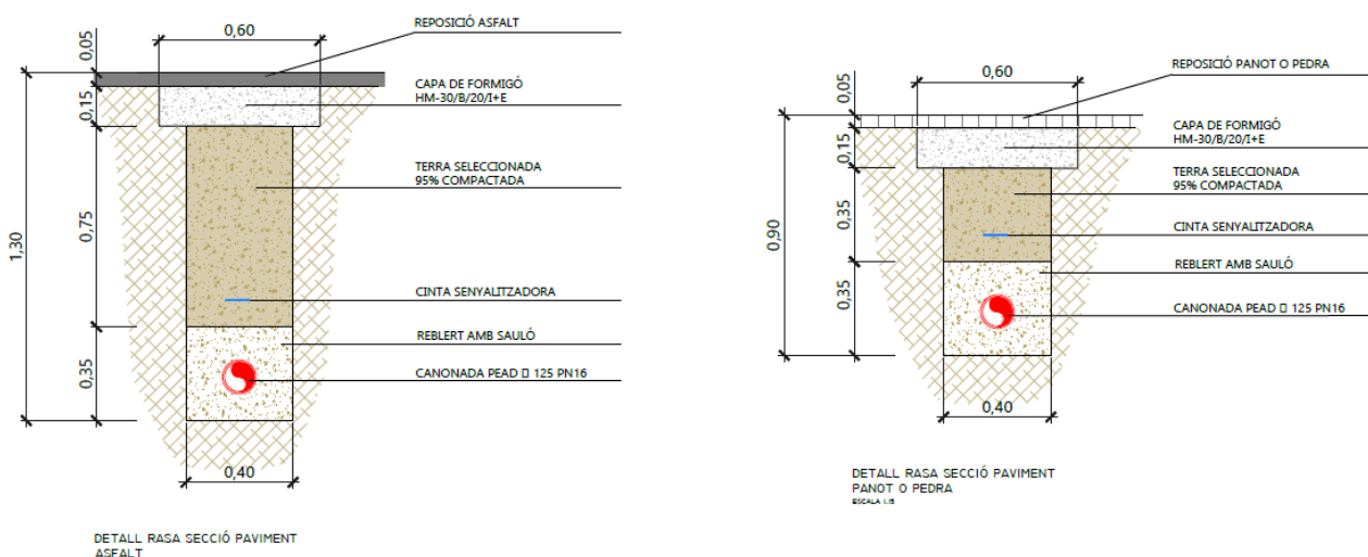
Figura 2: Detall rases projectades
