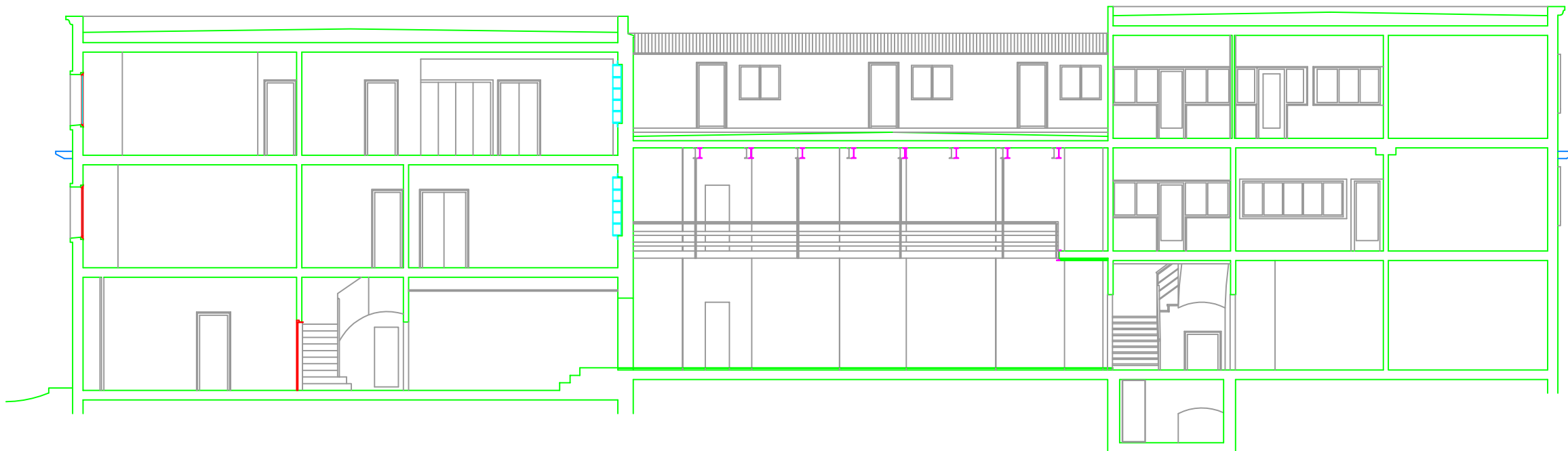
SECCIÓ A-A'
