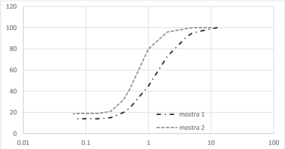
Corbes granulomètriques obtingudes
