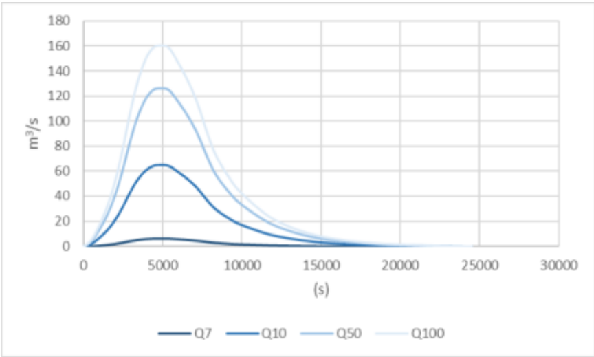
Figura 7. Hidrogrames de càlcul. Riera de Pineda.
