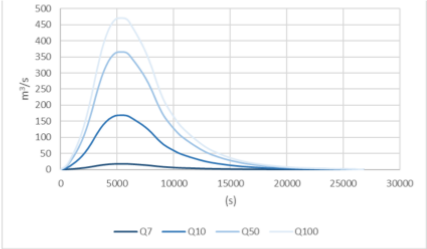
Figura 6. Hidrogrames de càlcul. Riera d'Arbúcies.
