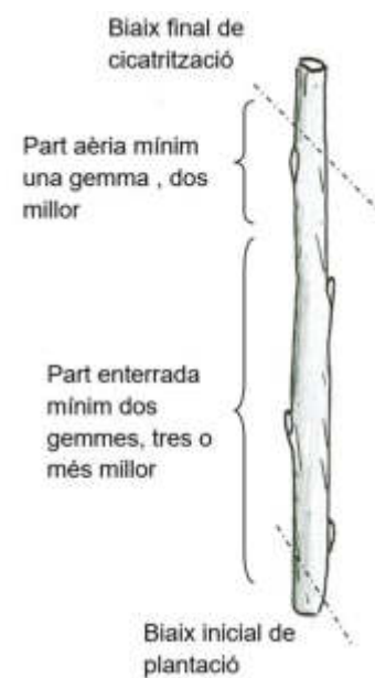
Preparació d'una estaca
