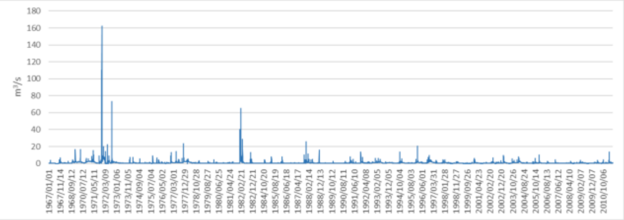
Figura 5. Cabals de l'estació d'aforament de Sant Feliu de Buixalleu (EA056) entre 1967 i 2011.
