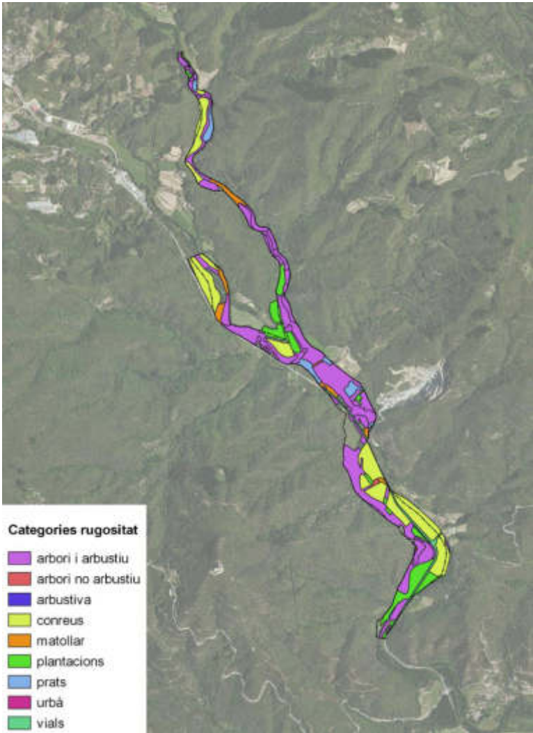
Figura 10. Categories de rugositat segons usos del sòl
