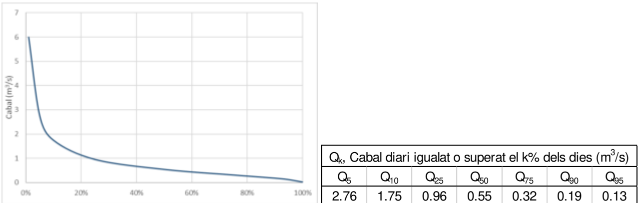
Figura 4. Corba de cabals classificats. Font: elaboració pròpia a partir de [5].
