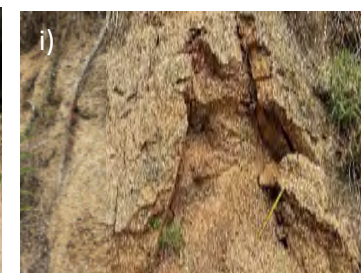
f) Granodiorita moderadament meteoritzada. g) Detall de la granodiorita, de gra mitjà a groller, travessada per algun filó de quars. h) Granodiorita moderadament meteoritzada i fissurada. i) Detall on s'observen diverses diàclasi que condicionen la progressió de la meteorització.
