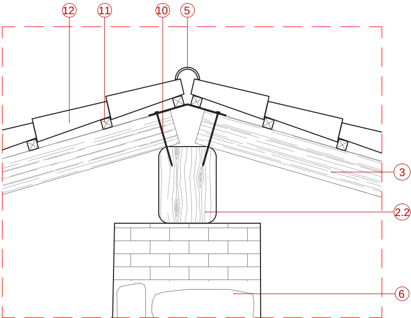
Detall 4
