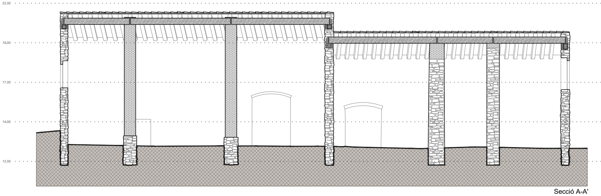
Secció A-A'
