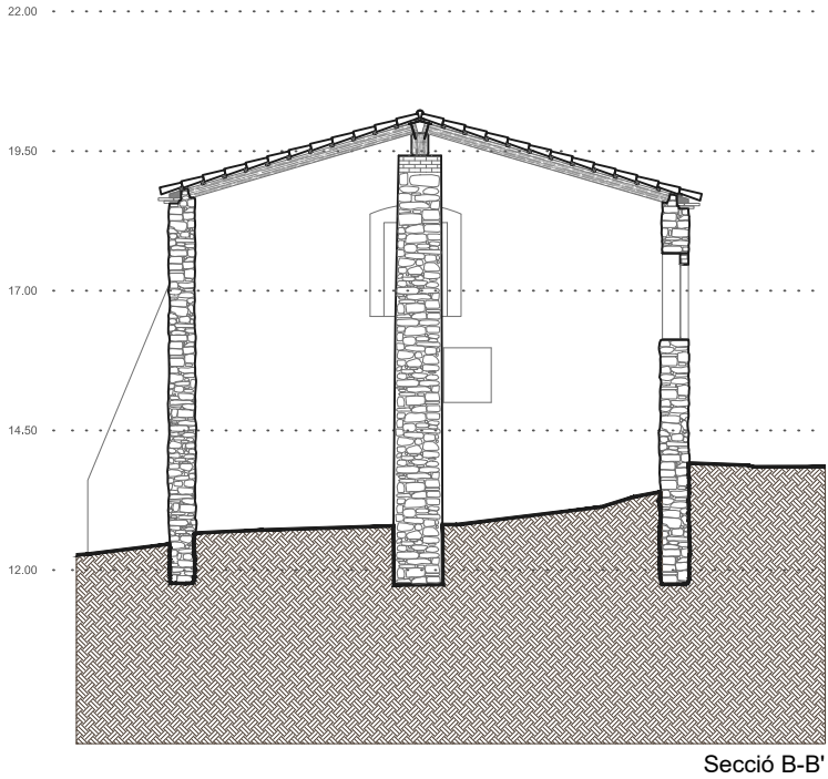
Secció B-B'
