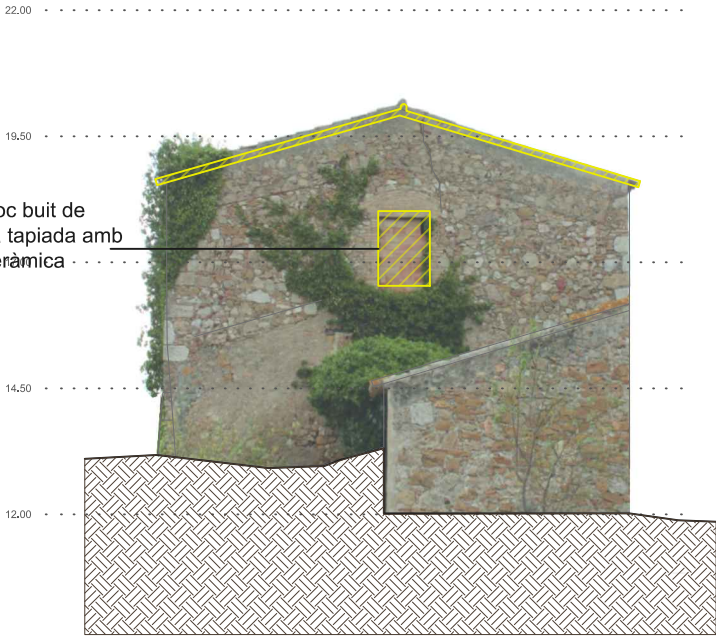
Alçat oest
