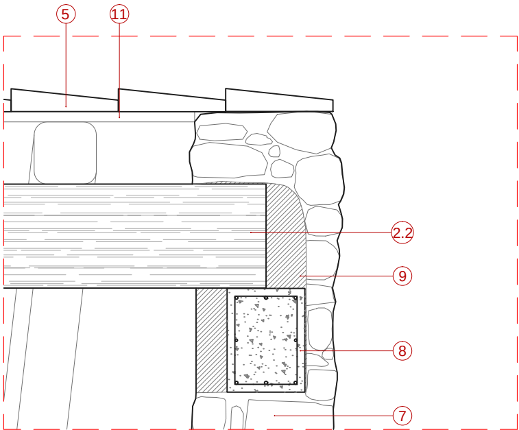
Detall 3
