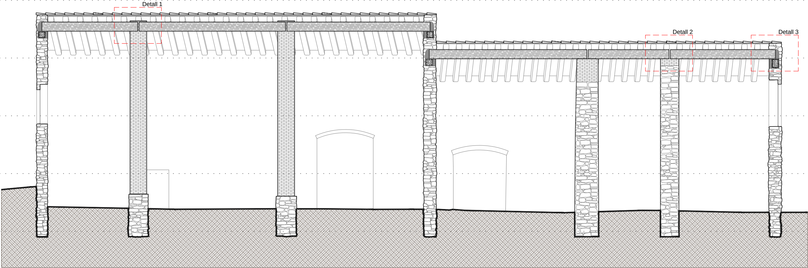
Secció A-A'
