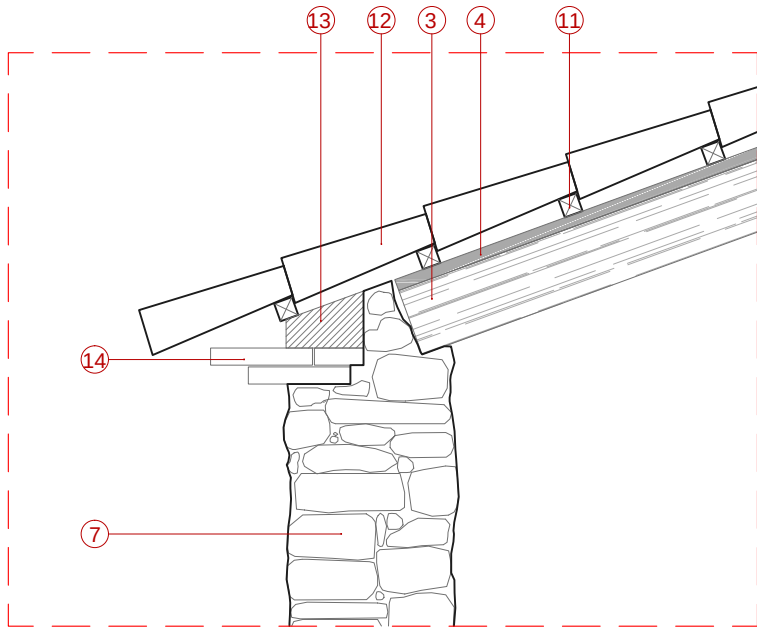
Detall 6
