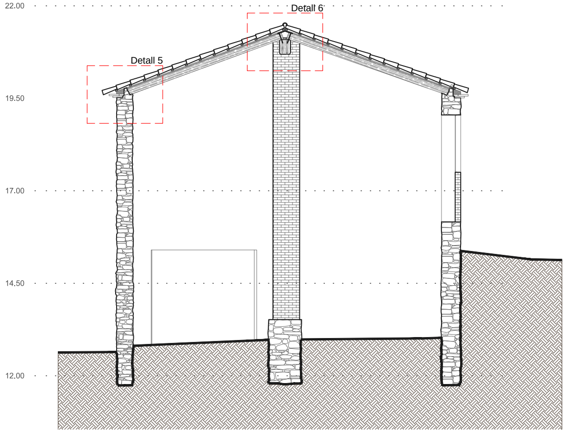
Secció C-C'
