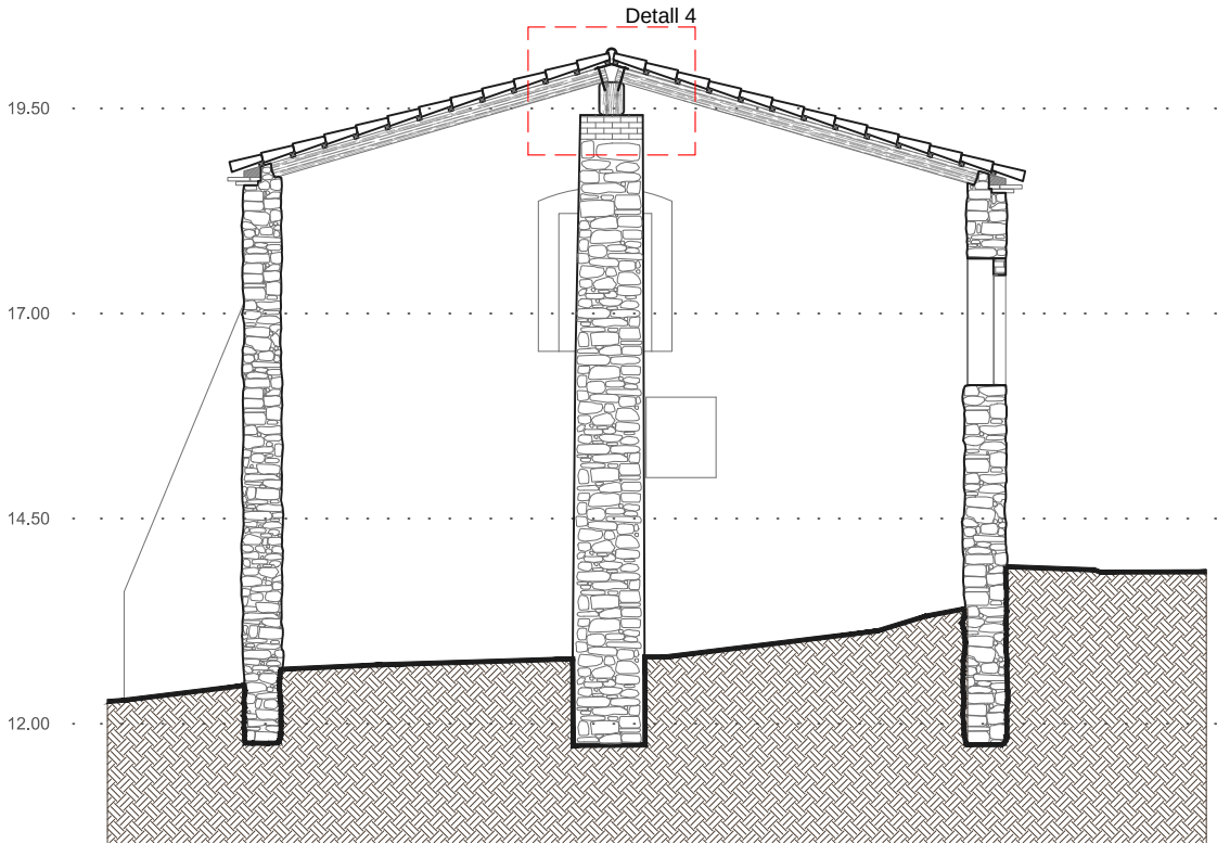
Secció B-B'
