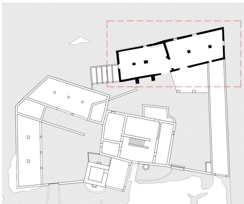
Planta de situació de l'àmbit d'intervenció en relació al Mas Vilanera
