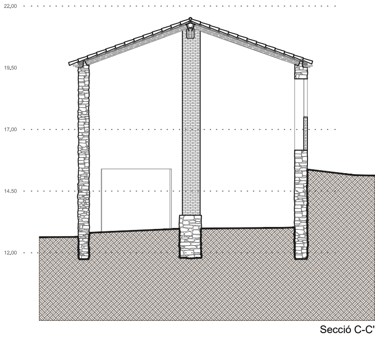
Secció C-C'
