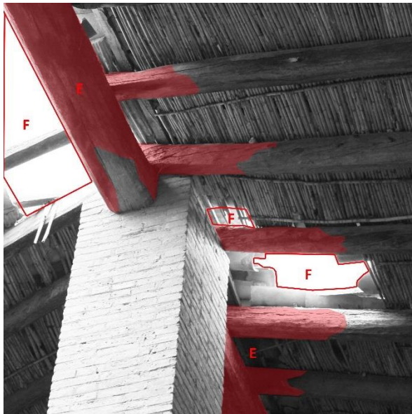
Vista de les patologies en els dos tipus de coberta dels edificis. E: degradació de les bigues principals i secundàries pels efectes de la humitat i la intempèrie. F: Desprendiment de teules degut al mal estat de l'entrebigat.
