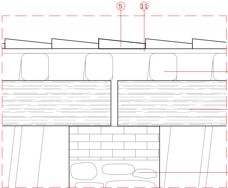
Detall 2
