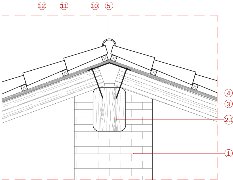
Detall 5
