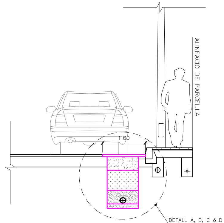
SECCIÓ DETALL DE RASA EN CALÇADA ESCALA 1/50
