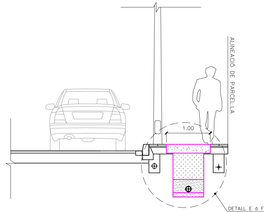
SECCIÓ DETALL DE RASA EN VORERA ESCALA 1/50
