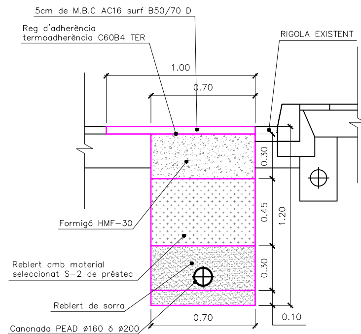
SECCIÓ DETALL A – SECCIÓ EN CALÇADA Ø160 i Ø200 ESCALA 1/25
