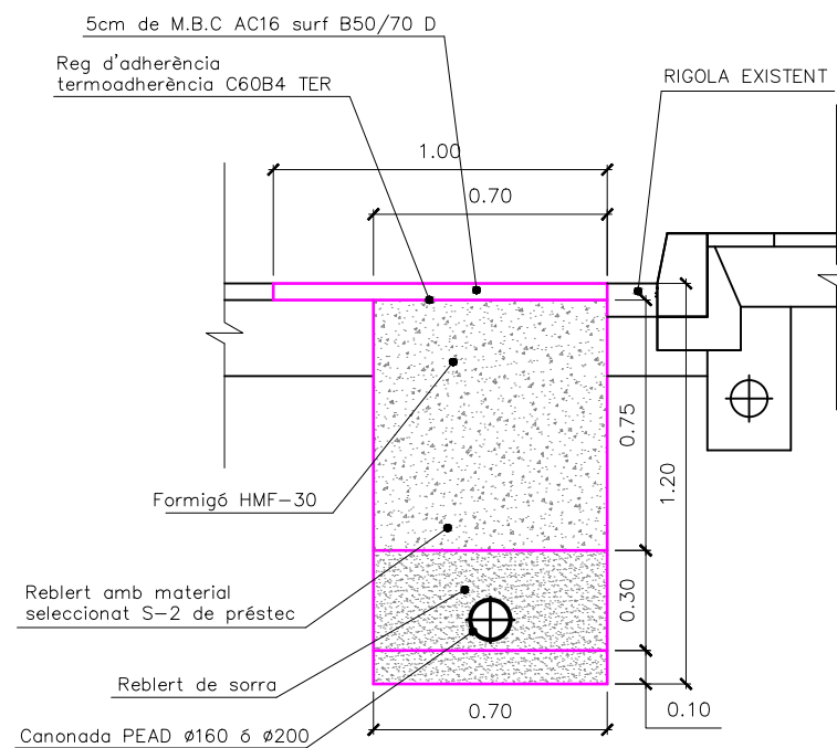
SECCIÓ DETALL B – SECCIÓ EN CREUAMENT DE CALÇADA Ø160 i Ø200 ESCALA 1/25
