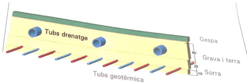
Esquema sobre el conjunt de sistema de geotèrmia, drenatge i gespa
