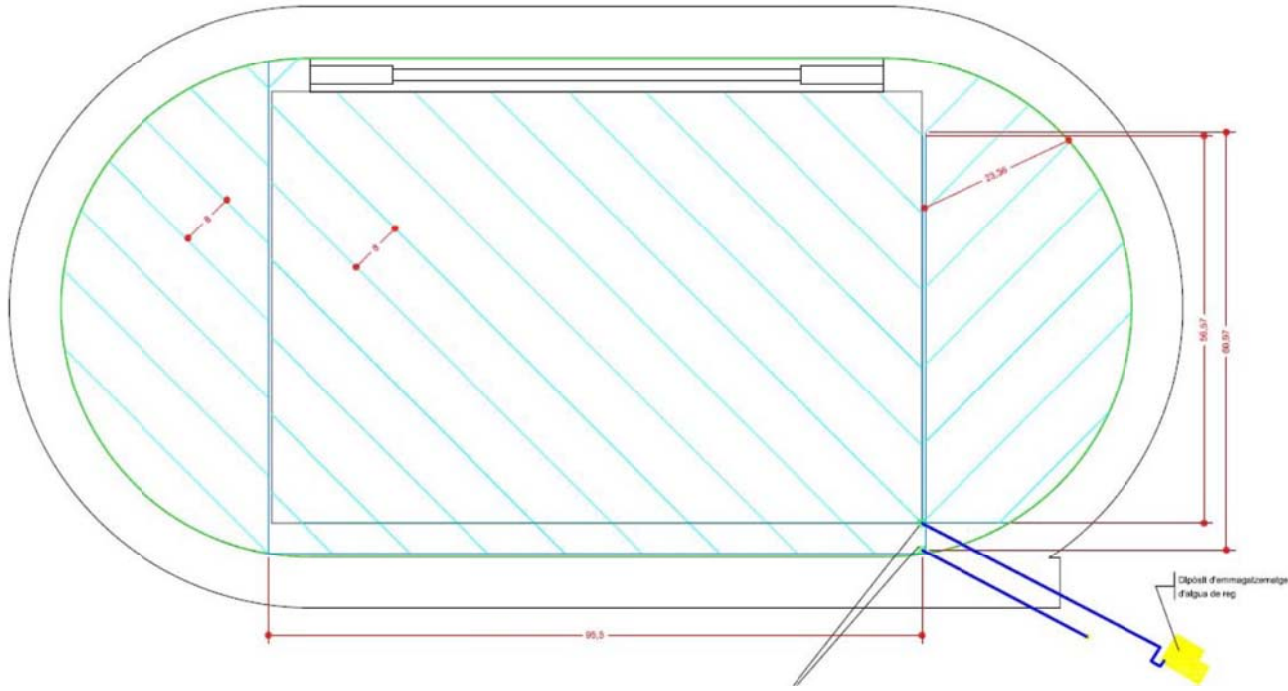
ESQUEMA XARXA DE DRENATGE
