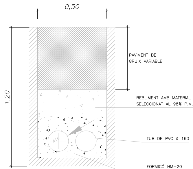
DETALL RASA TIPUS PER A CREUAMENT DE SERVEIS e. s/e
