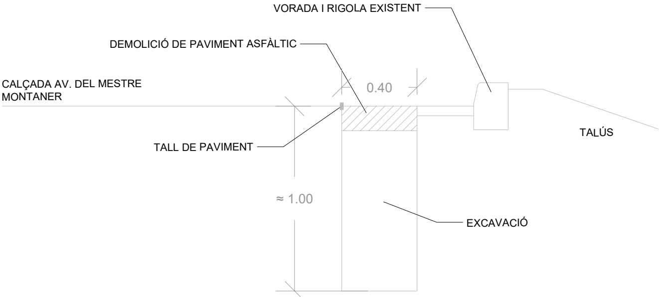
DETALL DEMOLICIÓ
