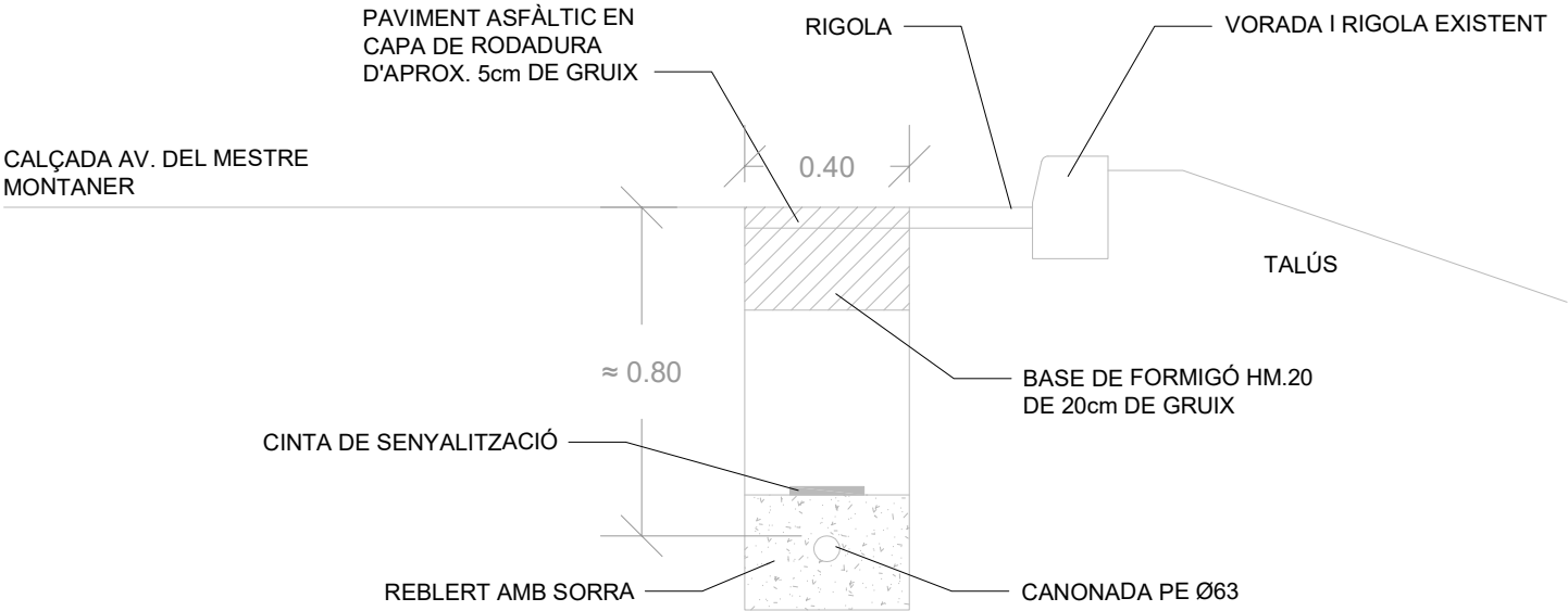
DETALL REPOSICIÓ
