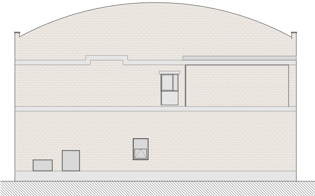
FAÇANA TRANSVERSAL
