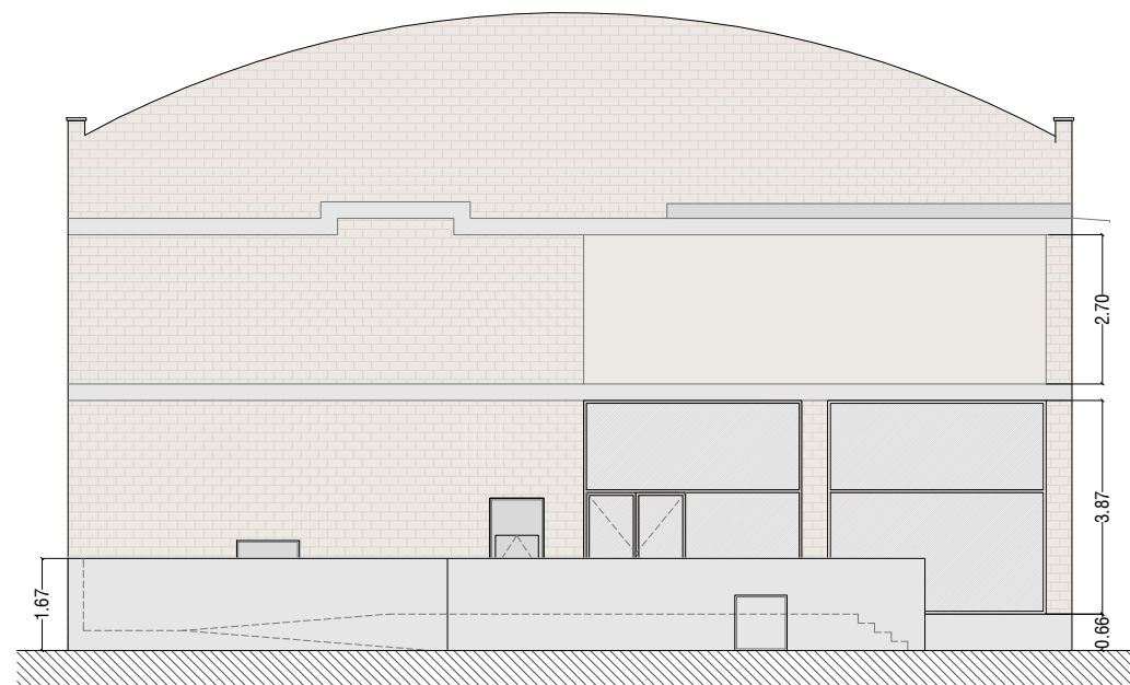
FAÇANA TRANSVERSAL
