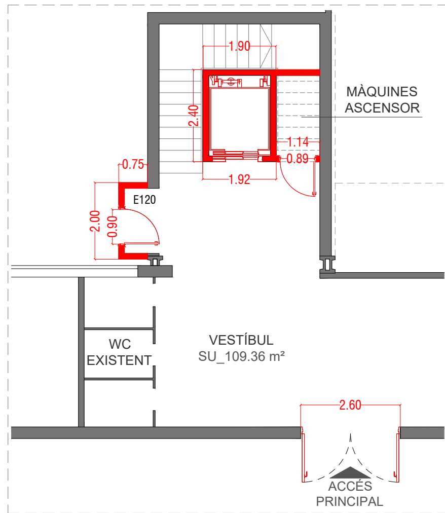
ZONA ASCENSOR - PLANTA BAIXA
