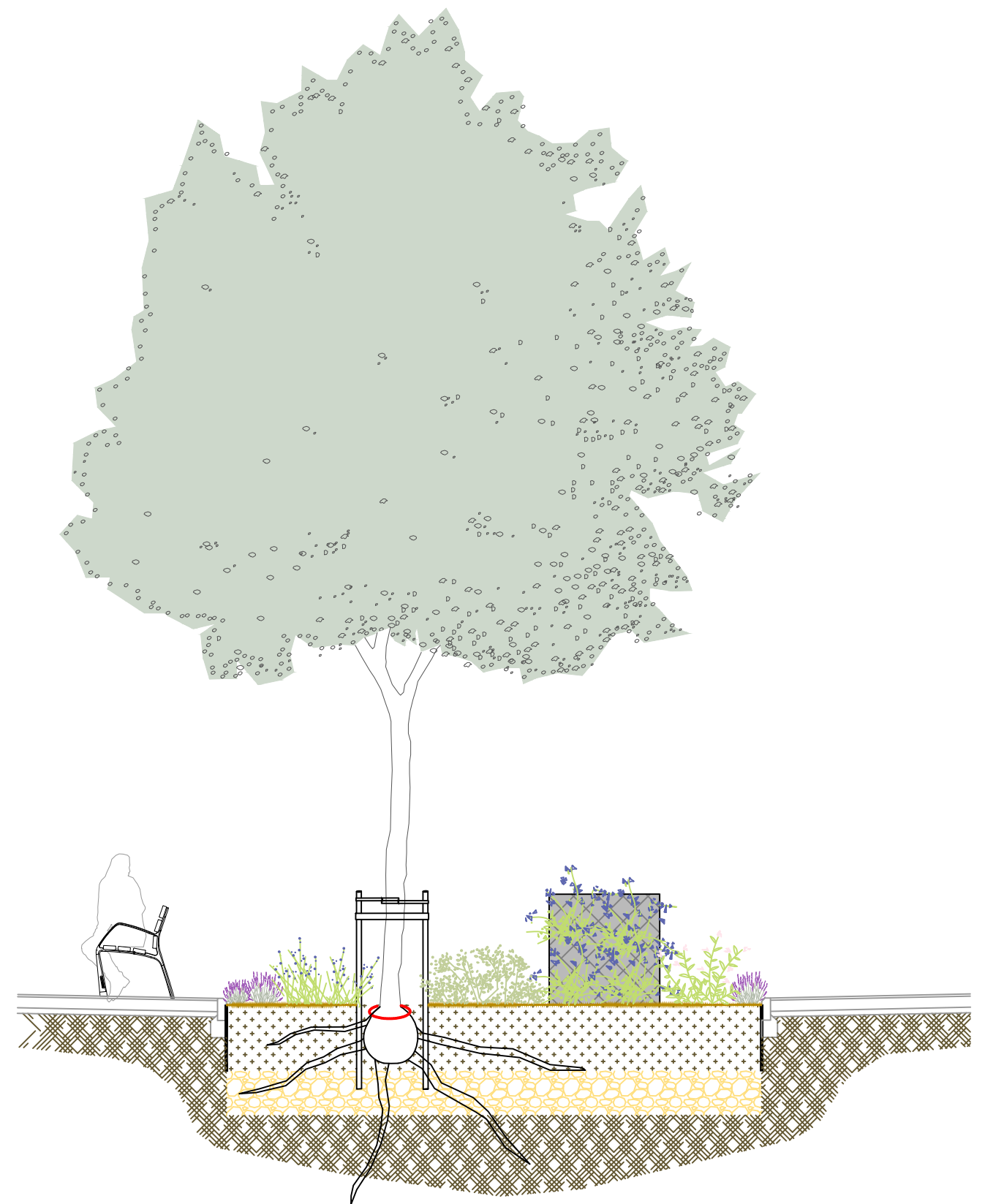
SECCIÓ CC'
