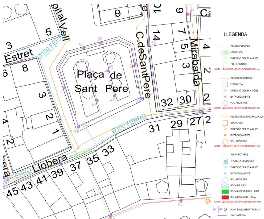
Plànol de les xarxes municipals existents de sanejament, aigua potable i enllumenat públic.
