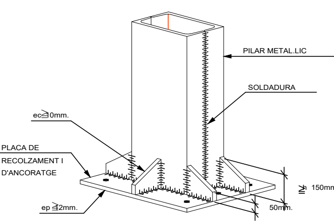
ARRENCADA DE PILAR EN FONAMENTS
