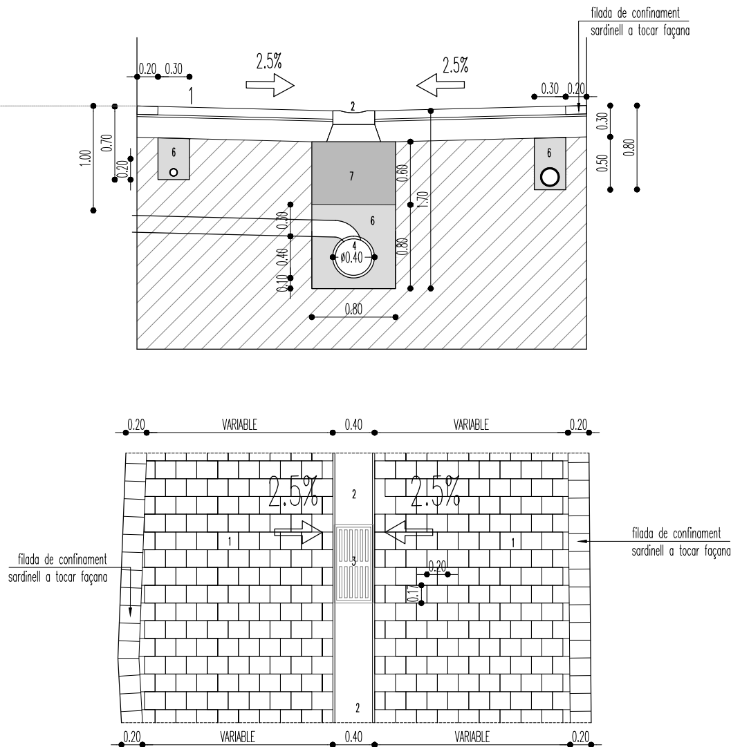
IMATGE – DETALL EMBORNAL INTEGRAT EN PAVIMENT
