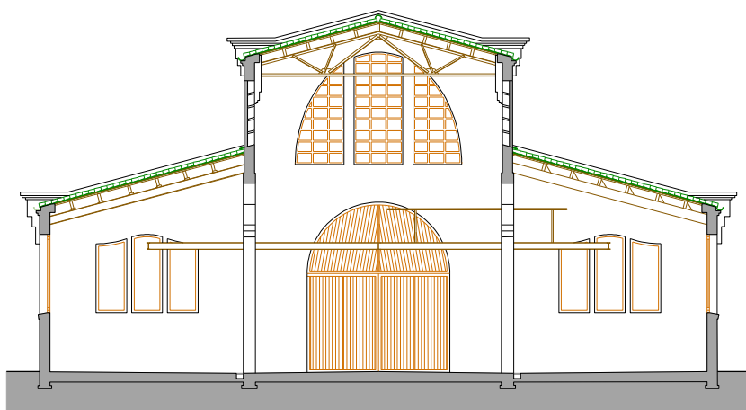
SECCIÓ A-A'
