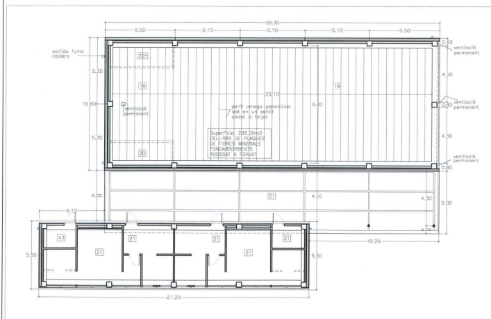
PLANTA CEL-RAS (tall cota 193.80 gimnàs, i cota 191.90 vestuaris)
