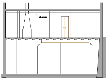
SECCIÓ B-B'
