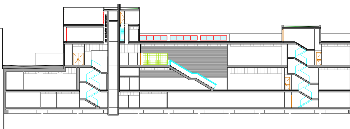
SECCIÓ H-H'
