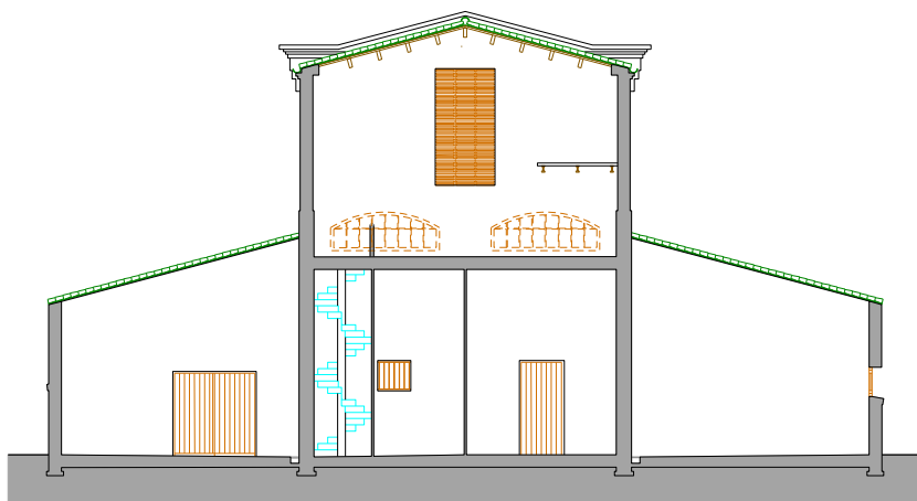
SECCIÓ B-B'
