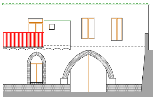
FAÇANA NORD
