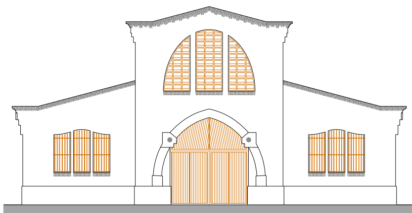
FAÇANA SUD-OEST
