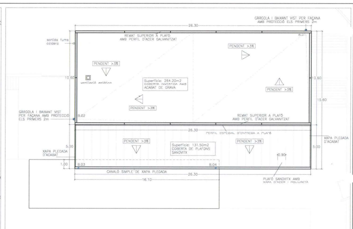
PLANTA COBERTA GIMNAS
