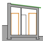
SECCIÓ D-D'
