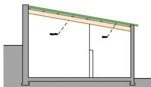
SECCIÓ B-B'
