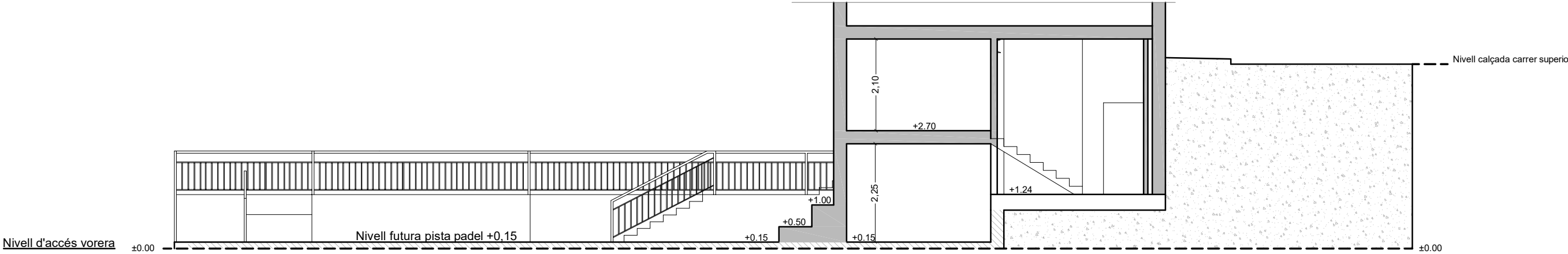
SECCIÓ CC
