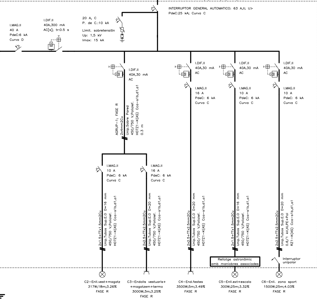
Cuadro General de Mando y Protección
