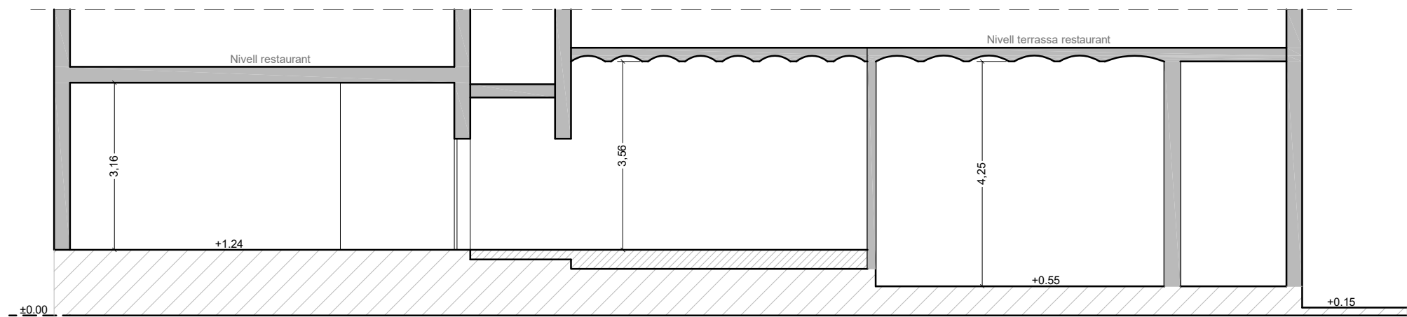
SECCIO AA
