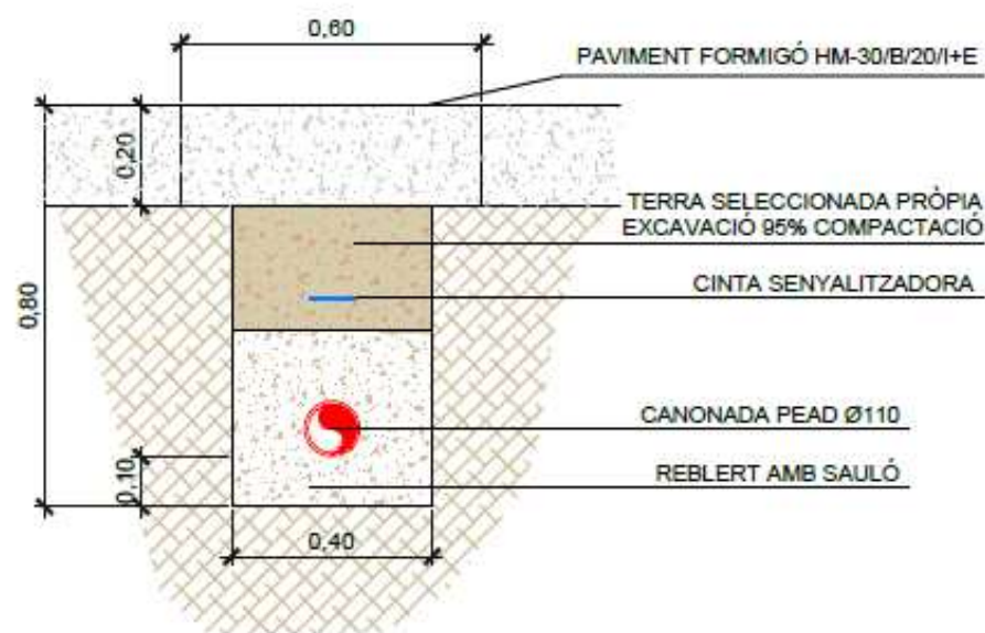
Figura 8. Detall tipus de rasa
