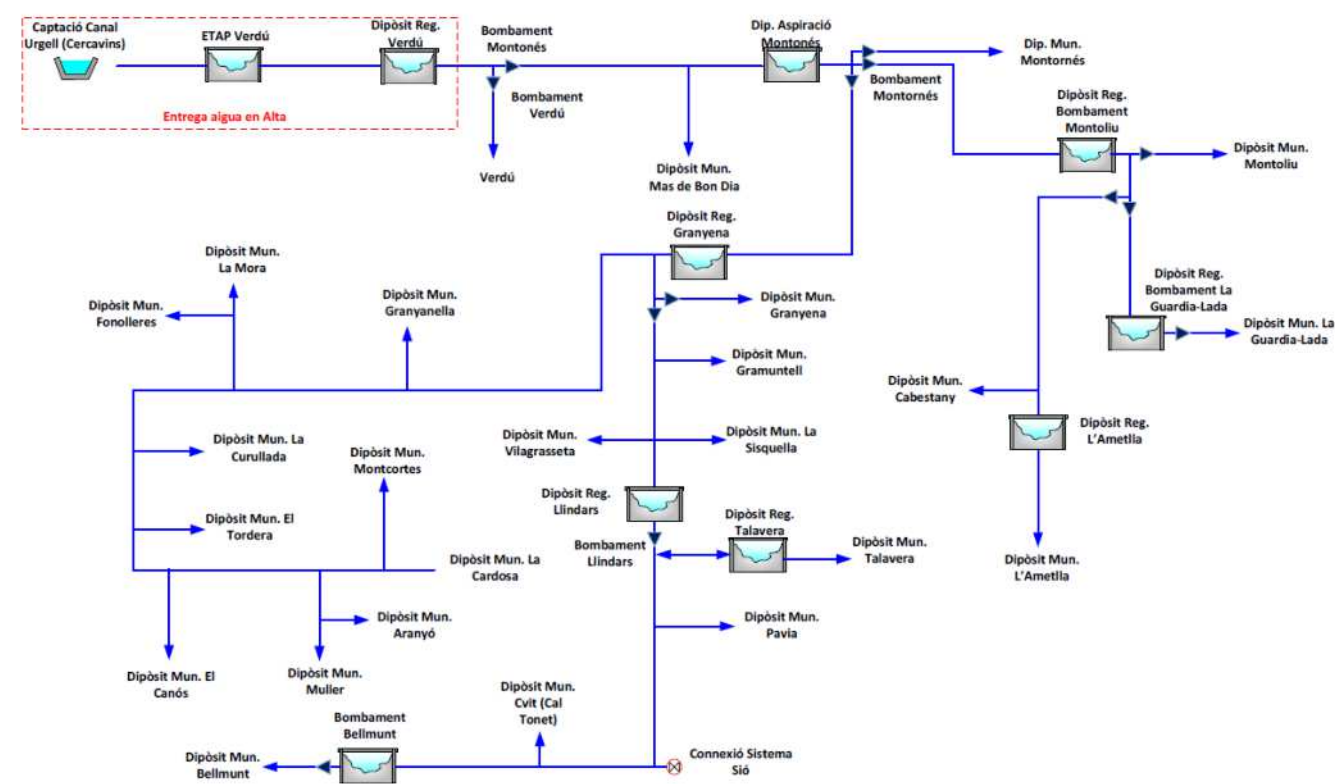
Figura 1. Esquema general xarxa abastament sistema Cercavins
