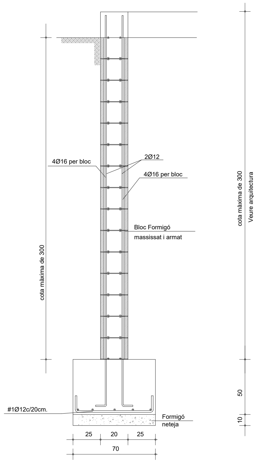
BLOC DE FORMIGÓ AMB FORJAT
