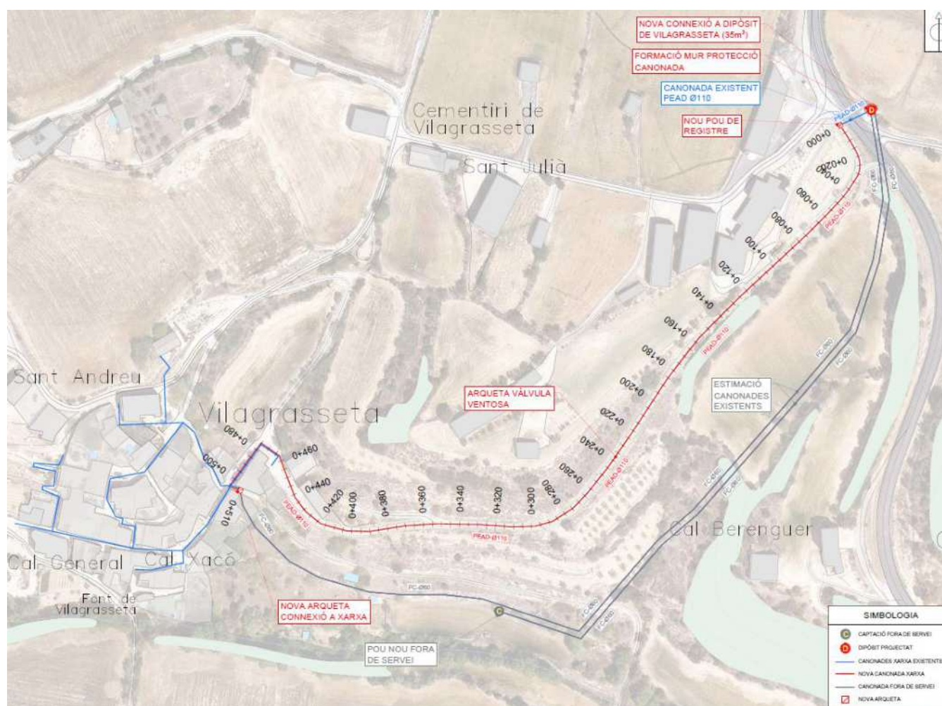
Figura 6. Traçat canonada projectada
