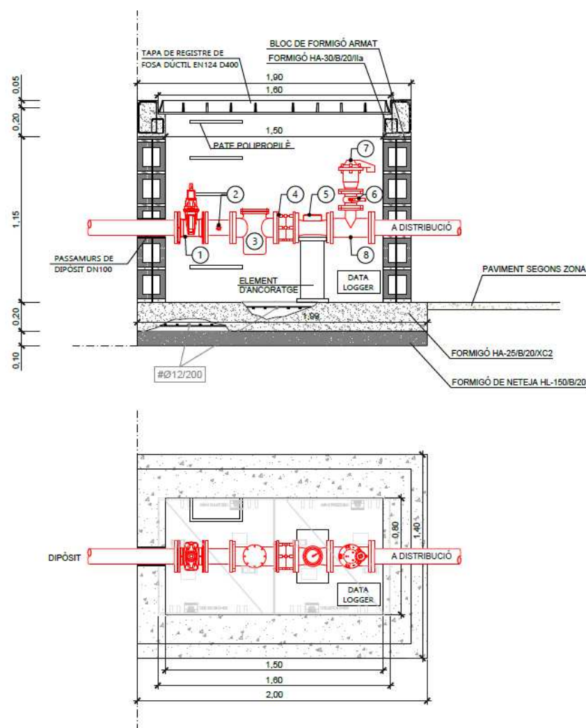
Figura 7. Arqueta tipus zona dipòsit
