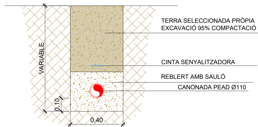
DETALL RASA PER CAMÍ DE TERRA
