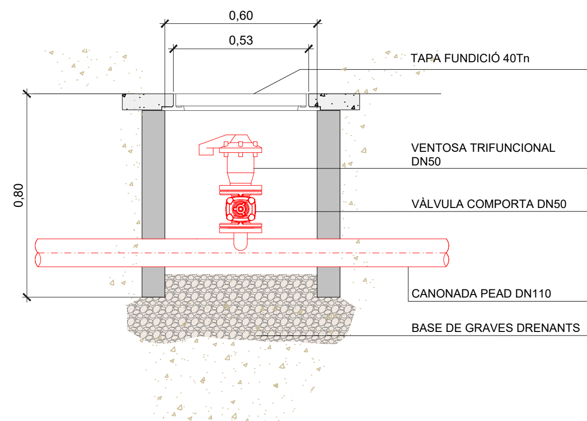
DETALL ARQUETA PER VÁLVULA VENTOSA
