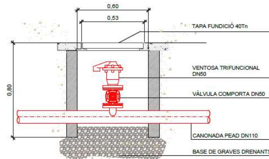
Figura 9. Detall arqueta per a vàlvula ventosa
