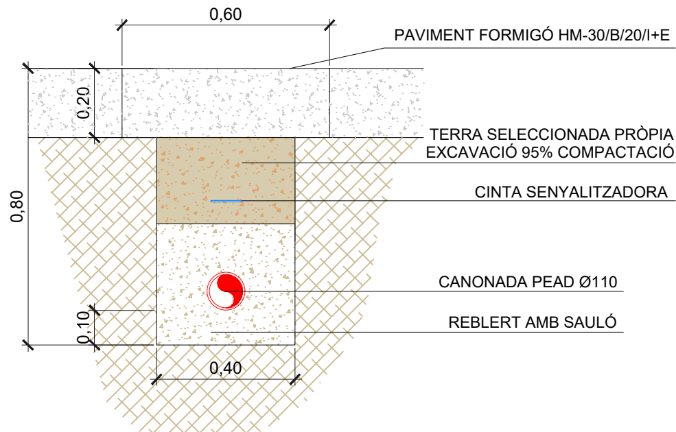
DETALL RASA PER PAVIMENT DE FORMIGÓ
