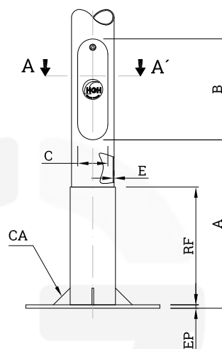
SECCIÓN A-A'
