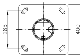
SECCION A-A'
