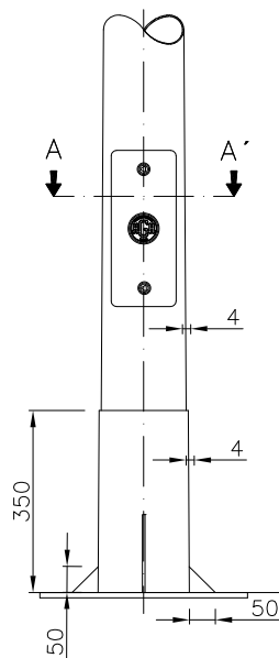
DETALLE 1
