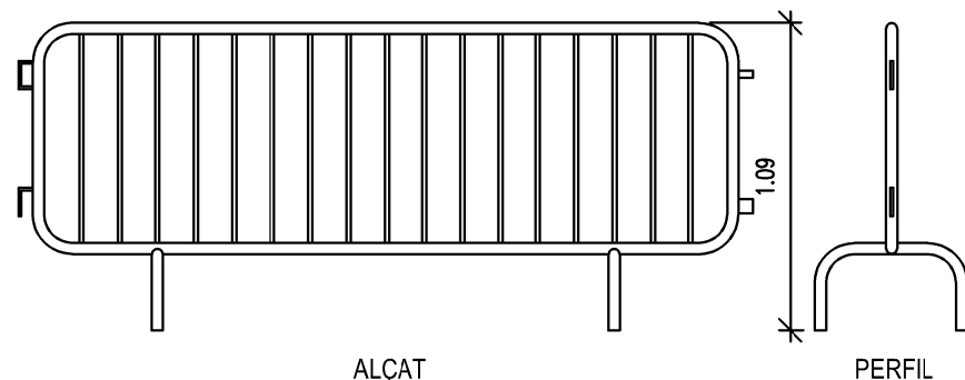
ALÇAT
