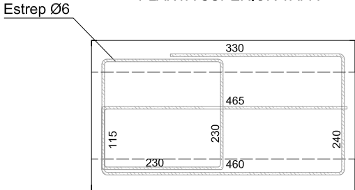
PLANTA SUPERIOR TAPA
