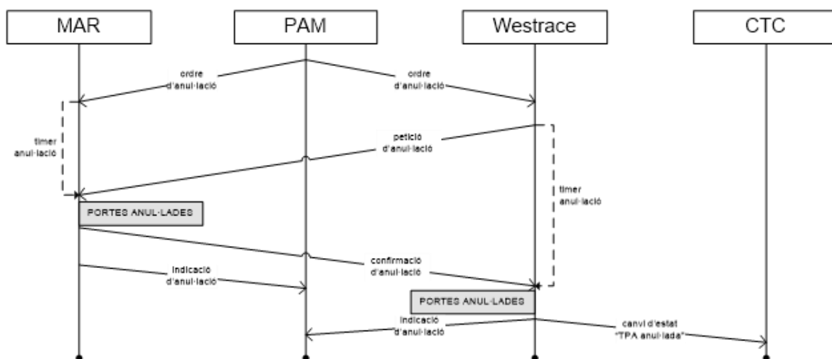
Figura 2. Diagrama d'anul·lació de portes des del PAM.
