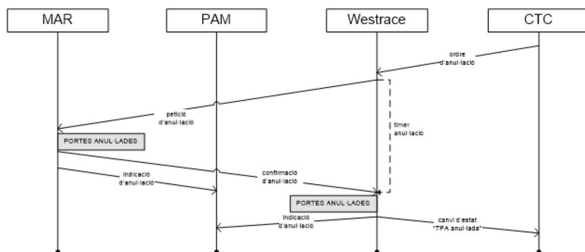
Figura 3. Diagrama d'anul·lació de portes des del CTC.
