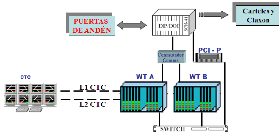
Figura 5. Arquitectura del sistema de senyalització de L11.
