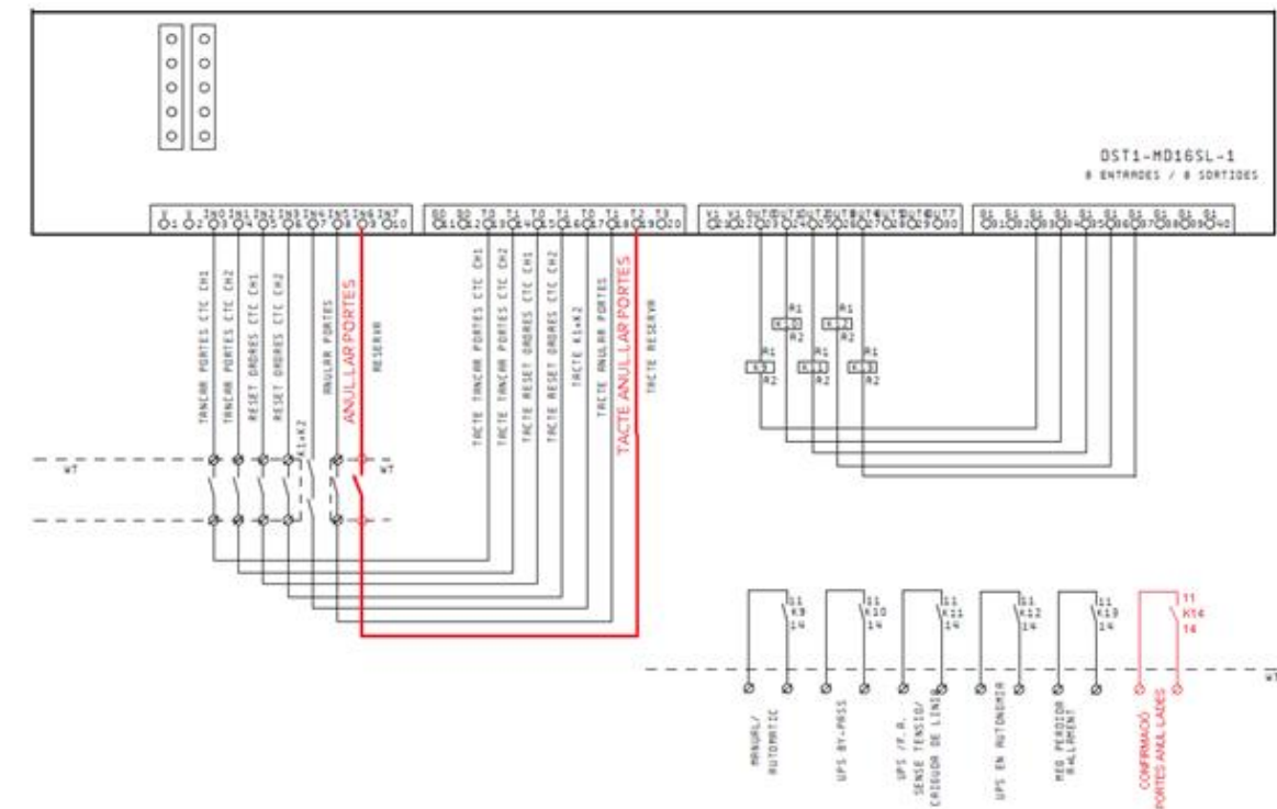
Figura 6. Cablejat previst per al MAR I/O.
