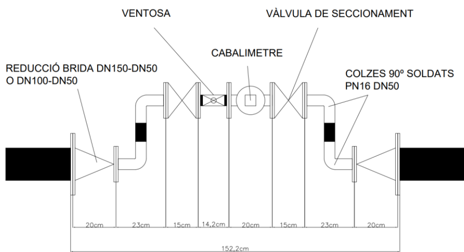
Figura 4. Configuració esquemàtica dels elements hidràulics d'una arqueta de sectorització.
