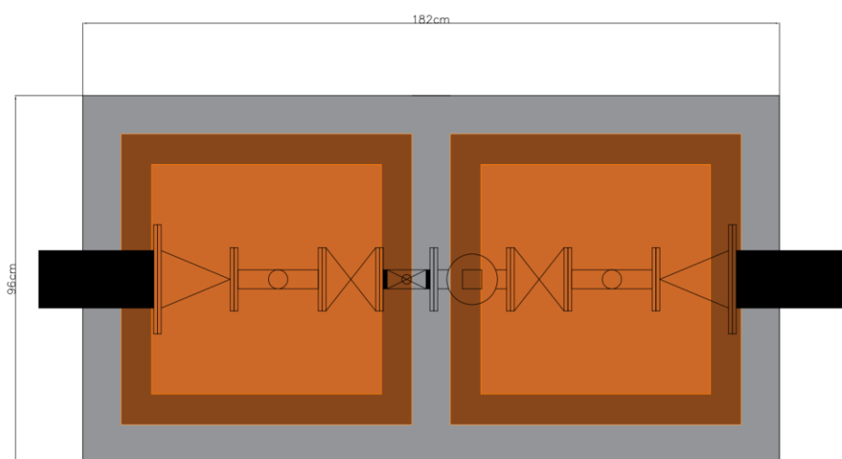
Figura 5. Dimensions de l'arqueta de sectorització.
