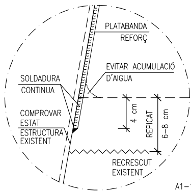
DETALL ARRENCADA PLATABANDA REFORÇ
