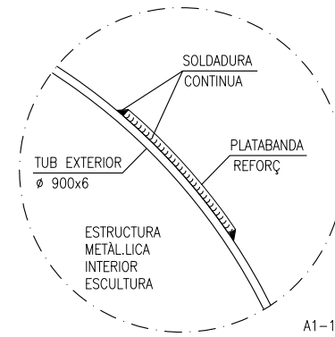
DETALL SOLDAT PLATABANDA REFORÇ
