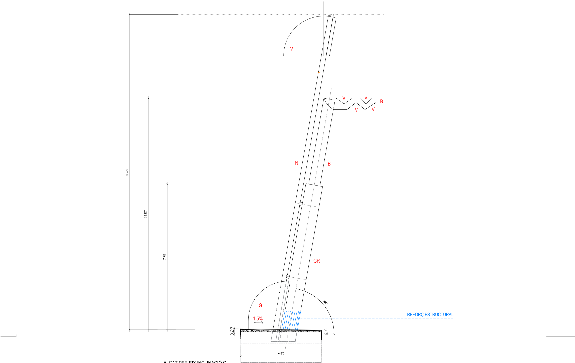
ALÇAT PER EIX INCLINACIÓ C
