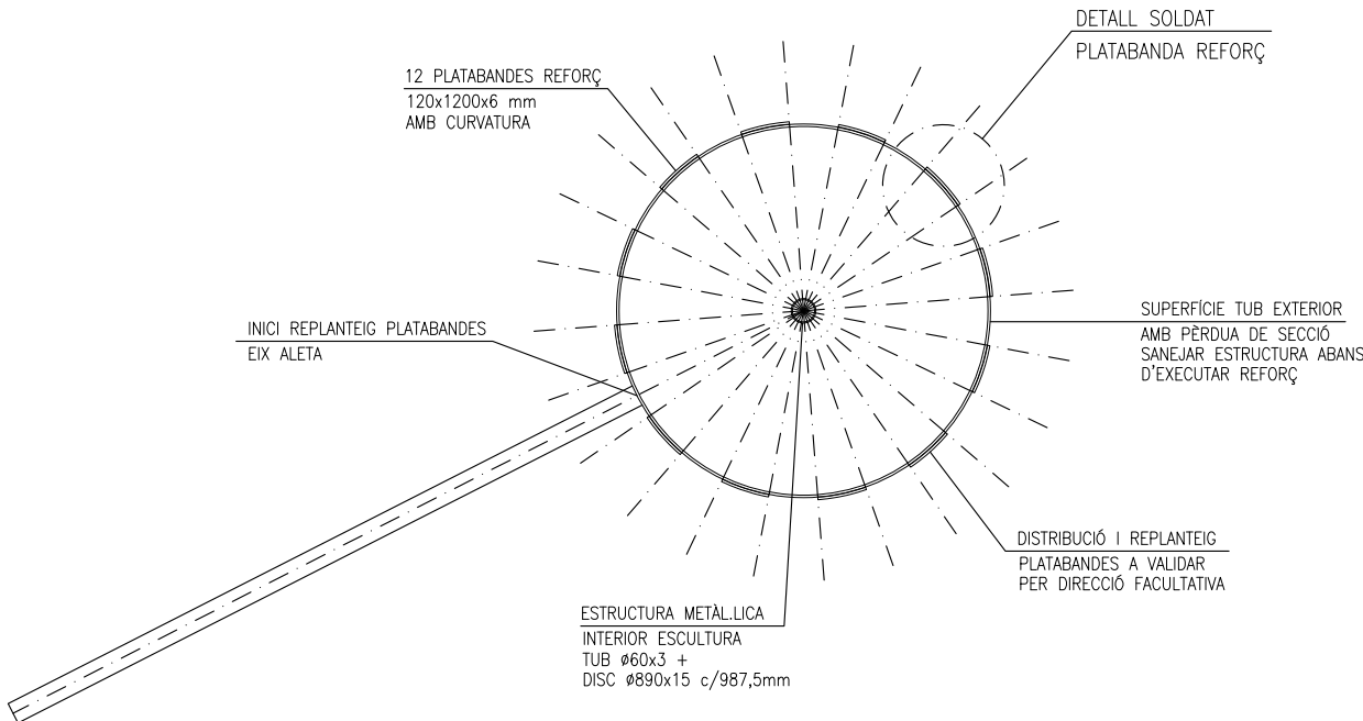
DETALL SOLDAT PLATABANDA REFORÇ
